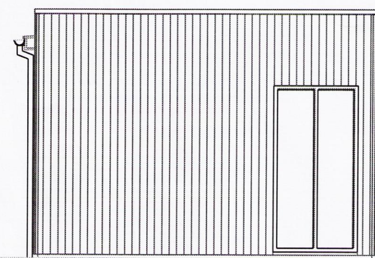
SUDVESTUR HLIÐ, 1:50
