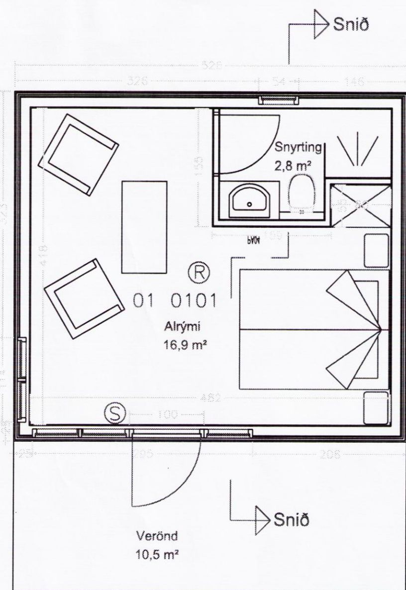
GRUNNMYND, 1:50
