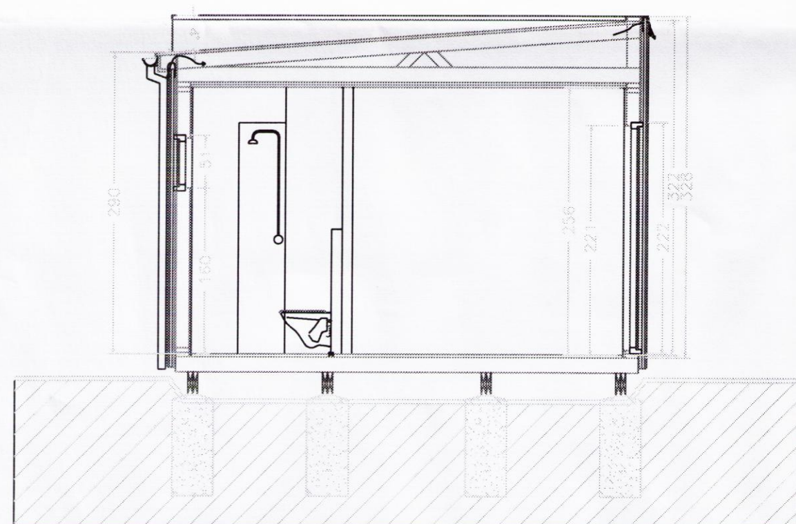
SNID A-A, 1:50
