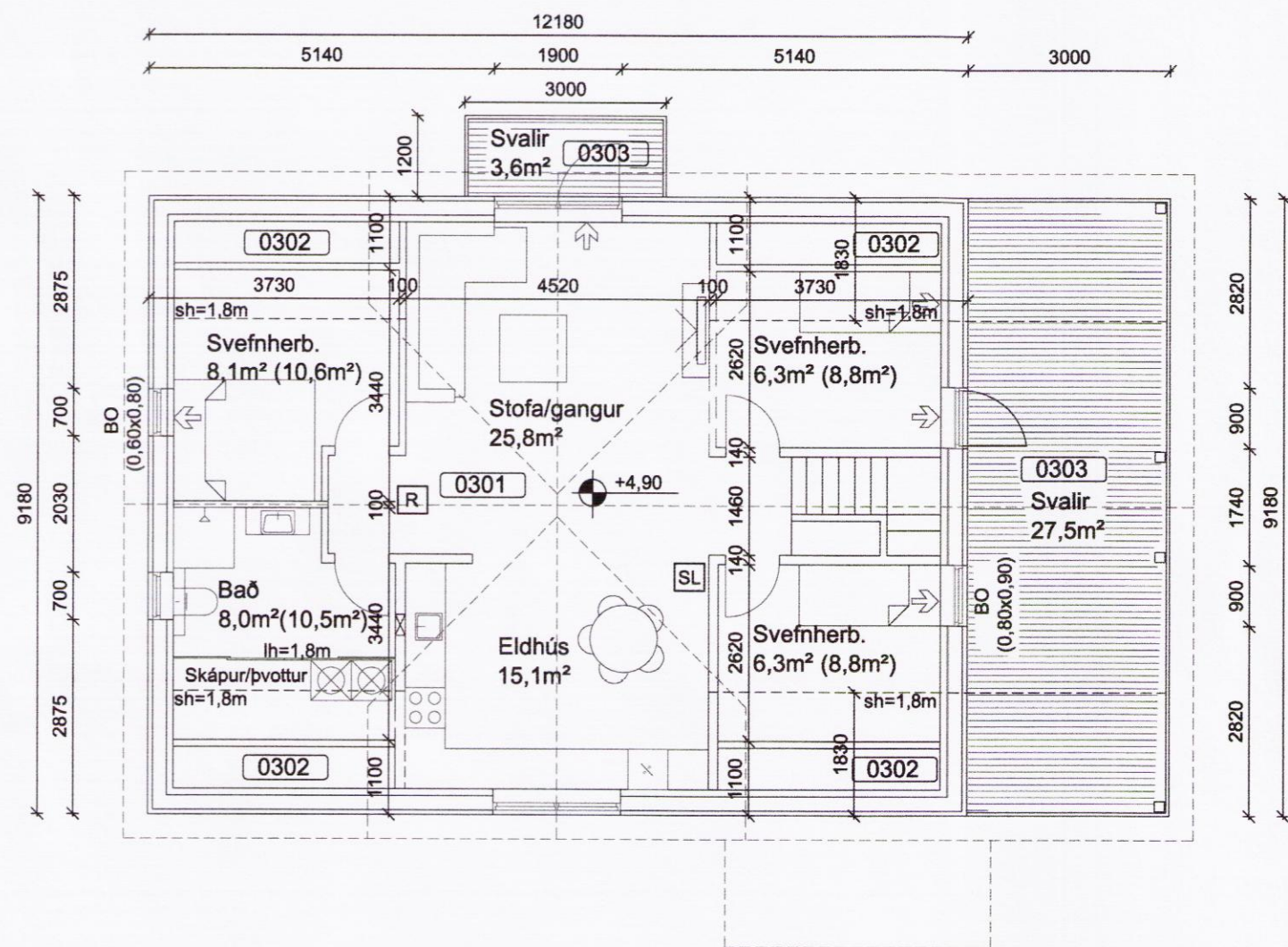
Grunnmynd ris hæðar eftir breytingu M 1:100
