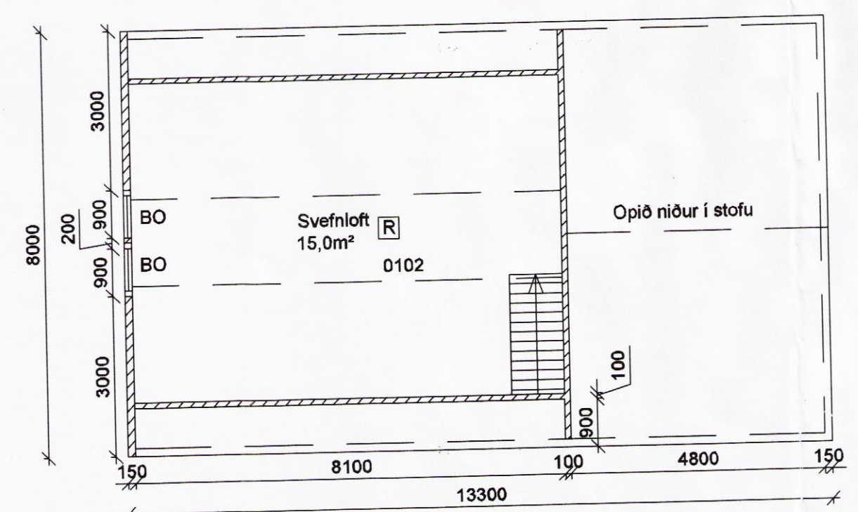
Grunnmynd svefnlofts mkv. 1:100
