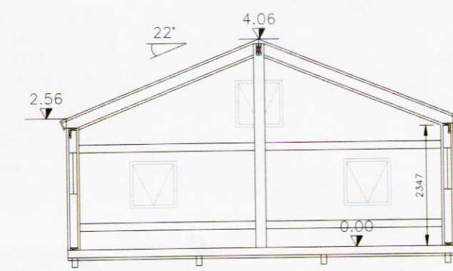
SNID 1 MKV. 1:50
