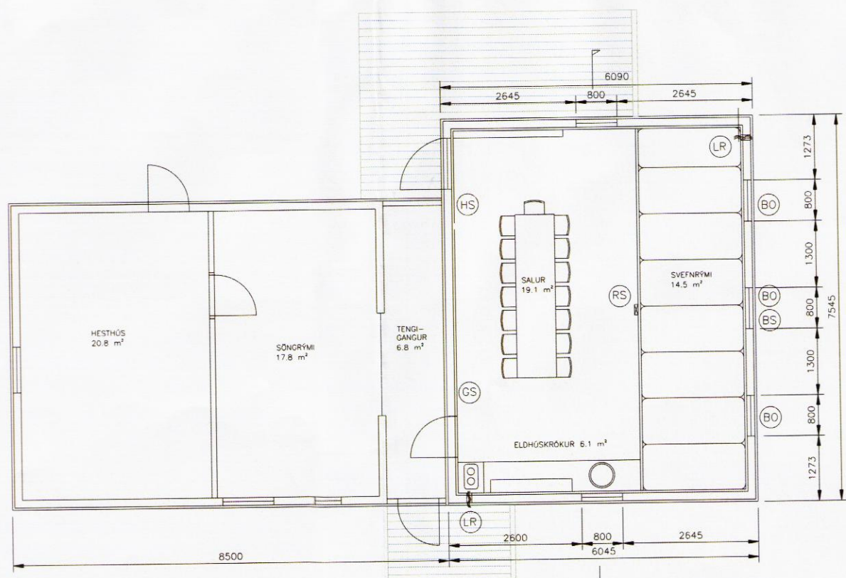
GRUNNMYND MKV. 1:50
