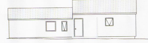
ÚTLIT SUÐAUSTUR MKV. 1:100
