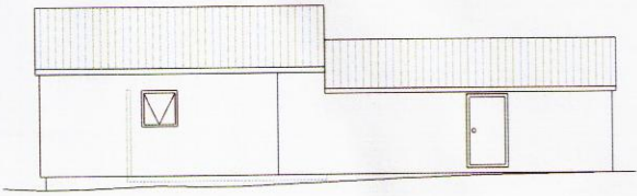
ÚTLIT NORÐVESTUR MKV. 1:100
