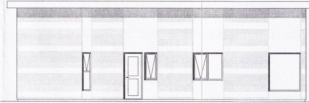
ÚTLIT NORÐVESTUR 1:100
