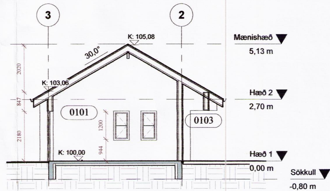
2 SKURÐUR Í VIÐBYGGINGU 1 : 100
