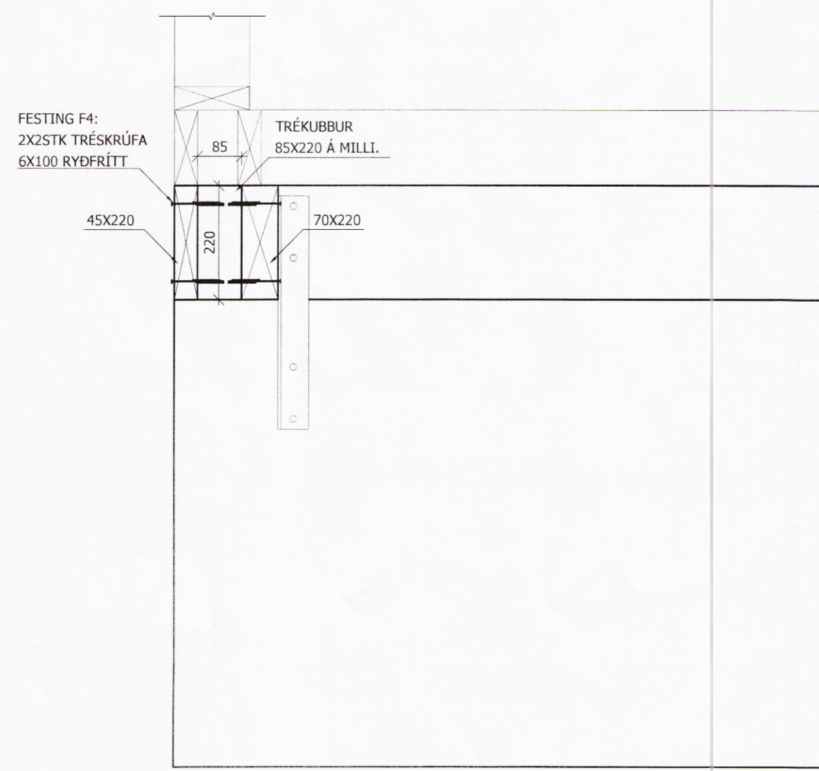
211 SNIÐ B Mkv 1:10
