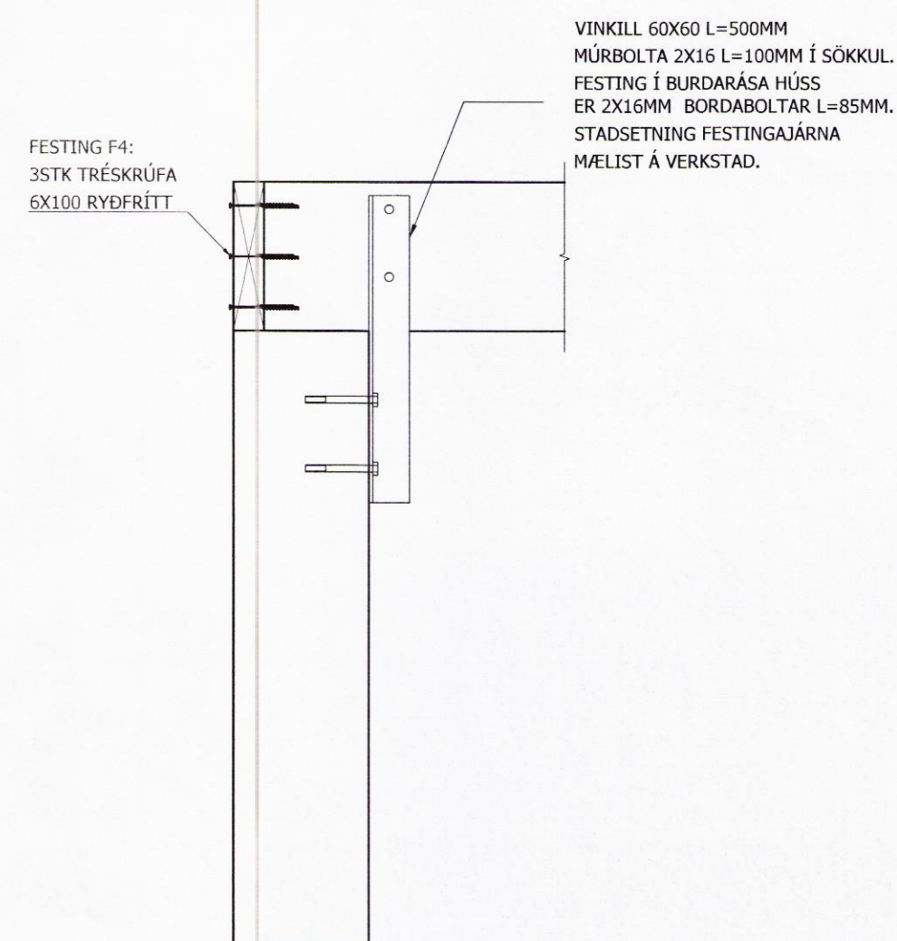
211 SNIÐ A Mkv 1:10
