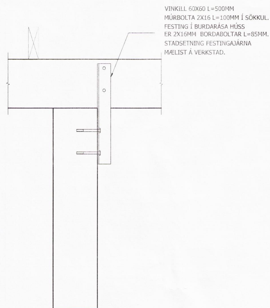
201 F1. FESTINGAR HÚSS VÍÐ SÖKKUL Mkv 1:10
