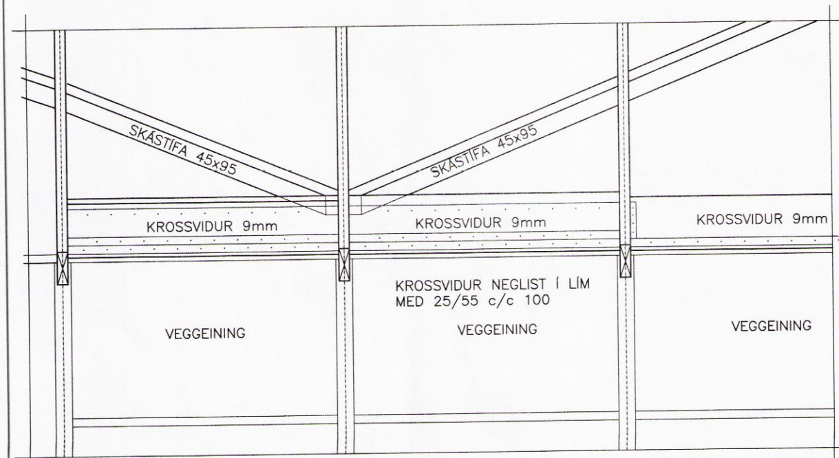
HLIÐARMYND MKV. 1:20
