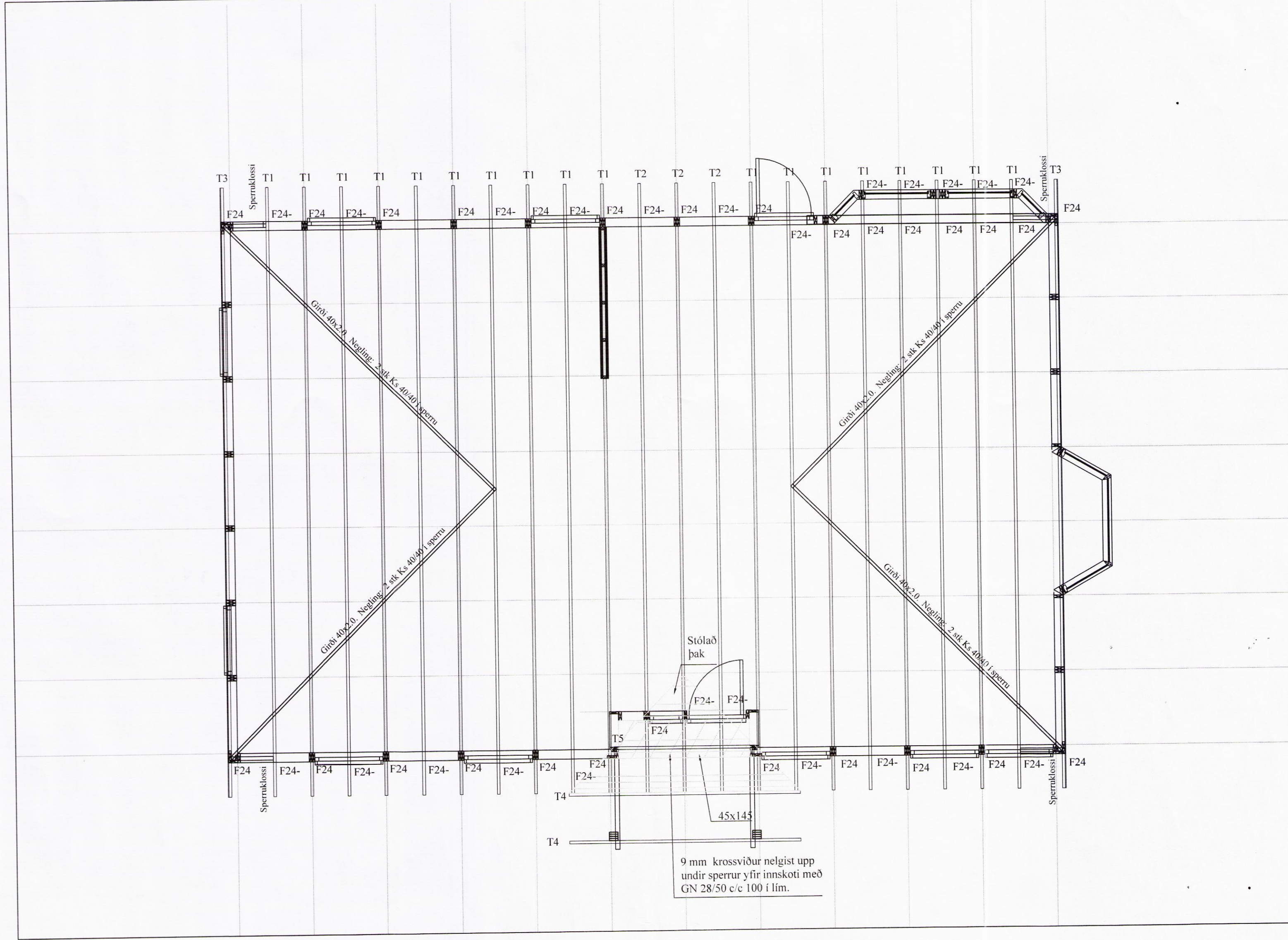
Grunnmynd þakplan MKV. 1:30
