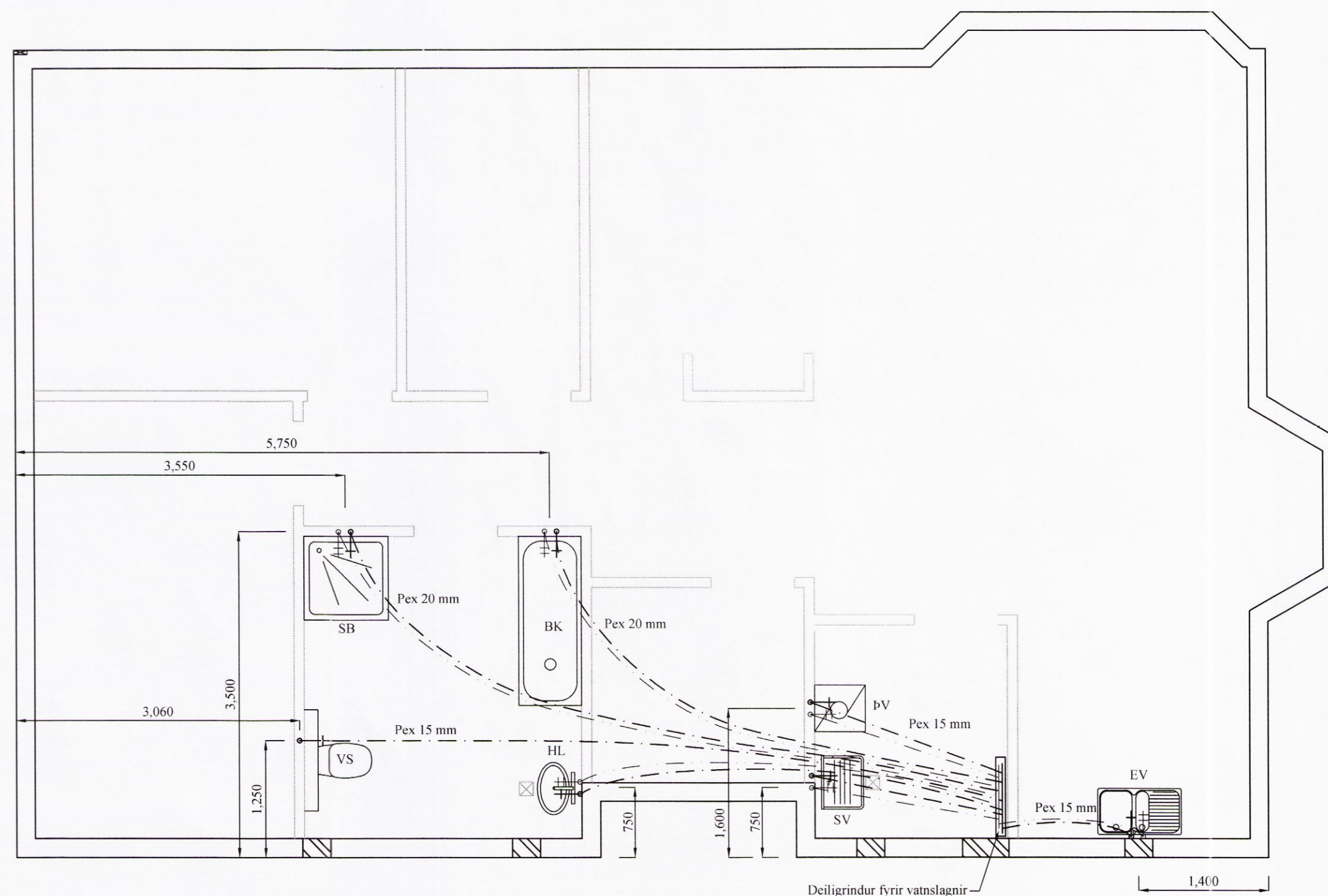
GRUNNMYND VATNSLAGNA Mkv. 1:50
