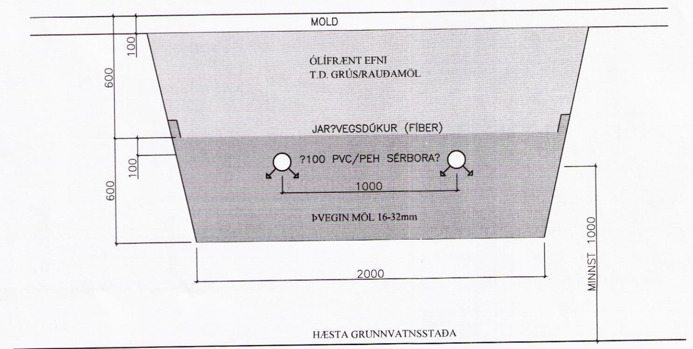
SNIÐ A SITURLÖGN Mkv. 1:20
