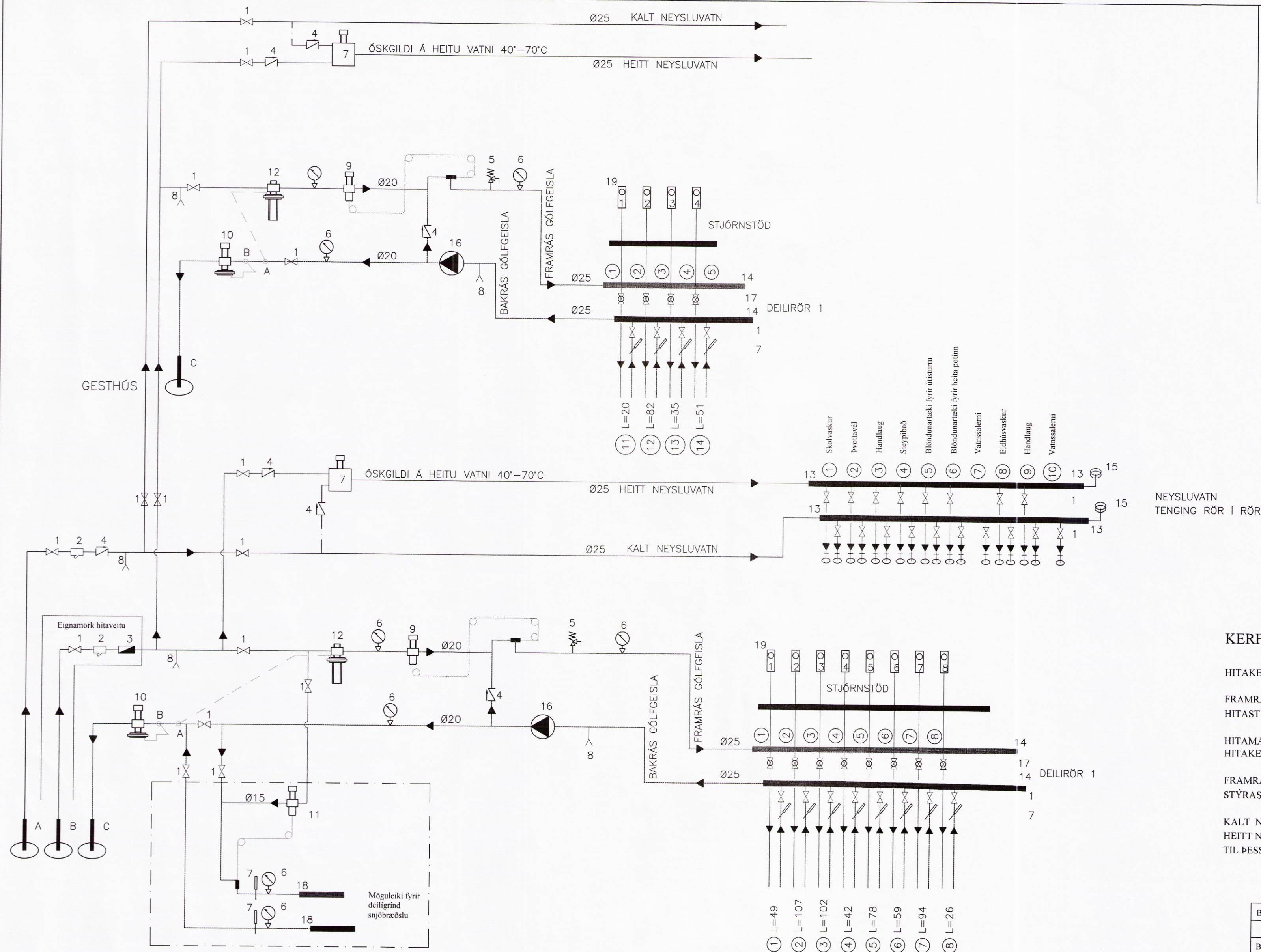
KERFISMYND HITÁ- OG NEYSLUVATNSKERFIS
