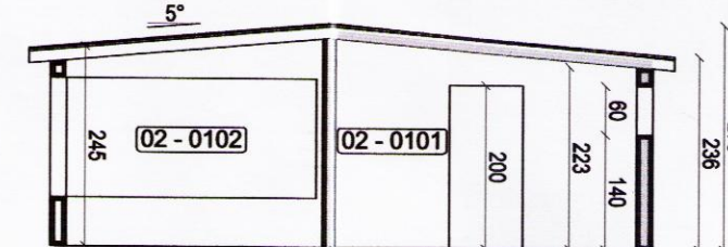
Sníð A-A Mkv 1:100
