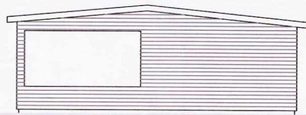
Austlæg hlið Mkv 1:100
