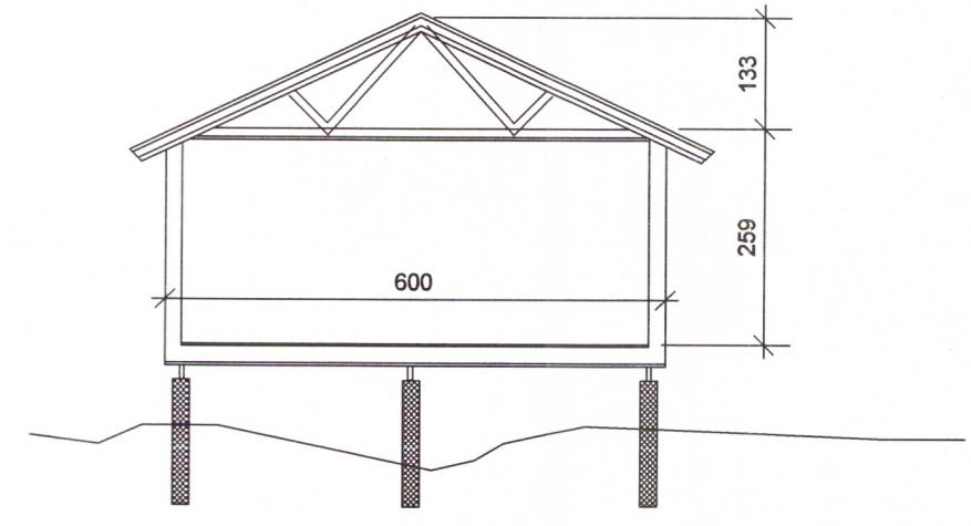
SNEIÐING A-A Mkv. 1:100
