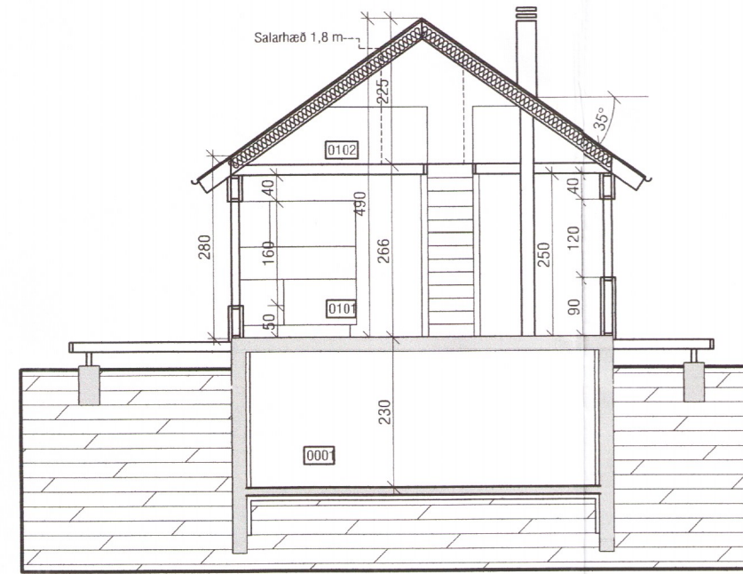
ÞVERSNIÐ A-A
