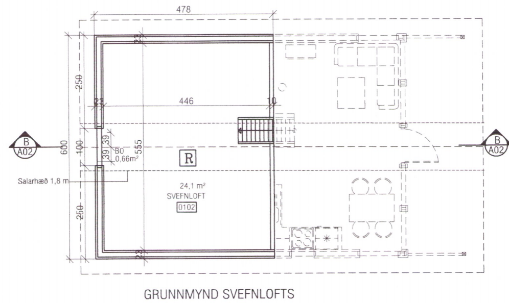
GRUNNMYND SVEFNLOFTS
