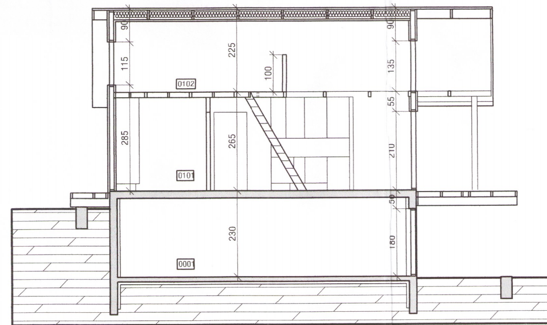
LENGDARSNÍÐ B-B
