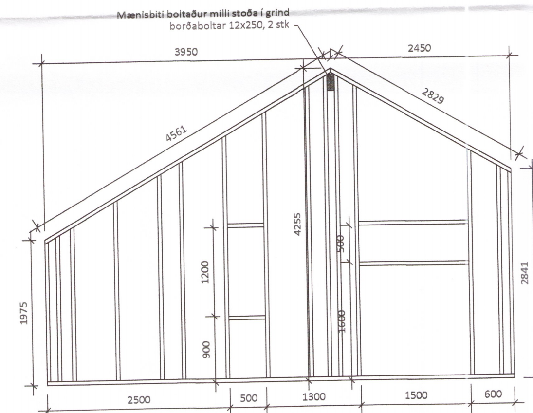
GRIND 2 Mkv. 1:50
