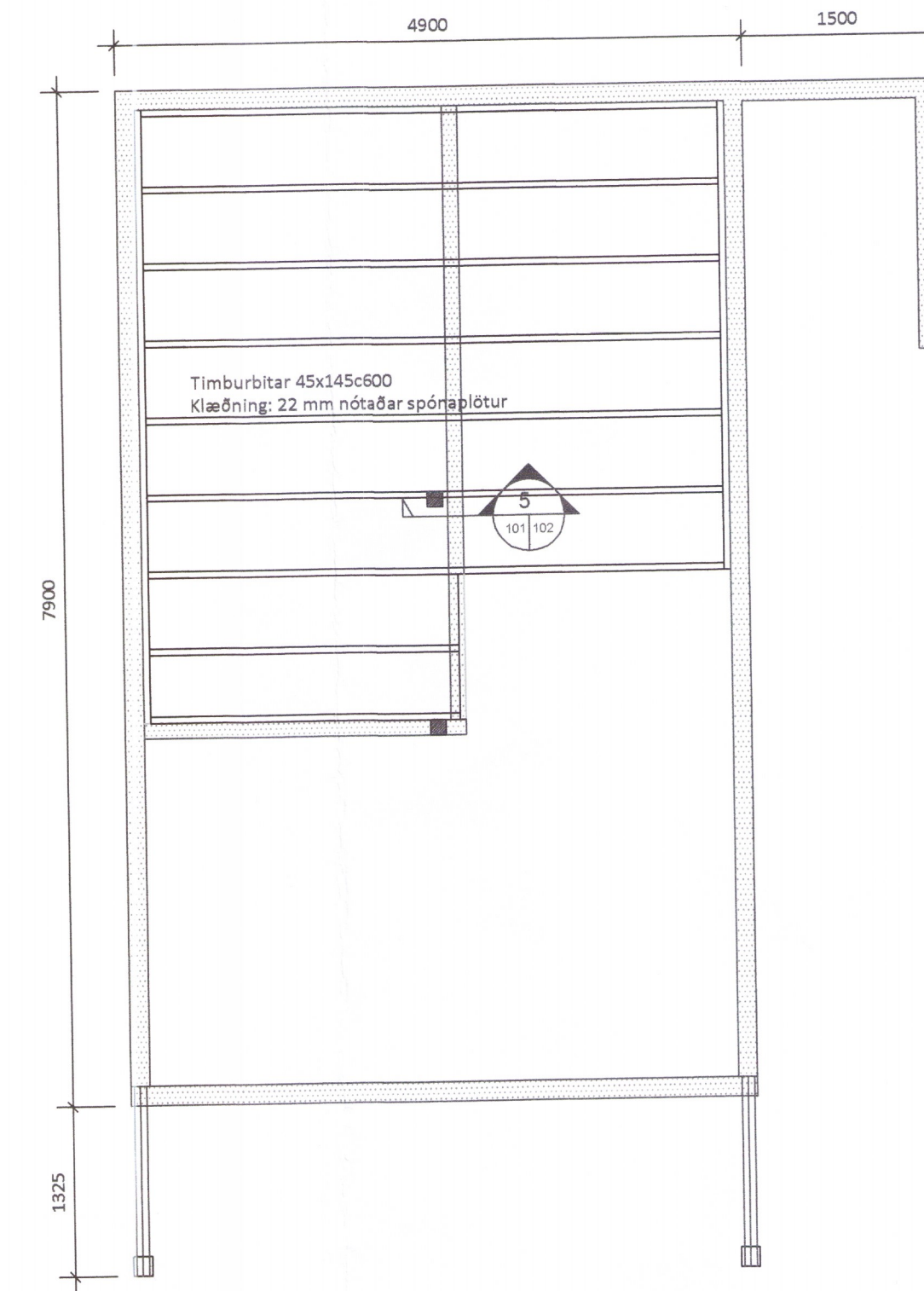
GRUNNMYND-MILLIGÓLF Mkv. 1:50
