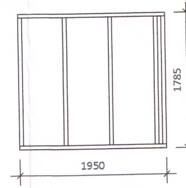
GRIND 3 Mkv. 1:50
