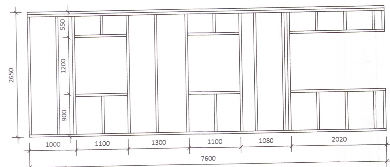
GRIND 1 Mkv. 1:50
