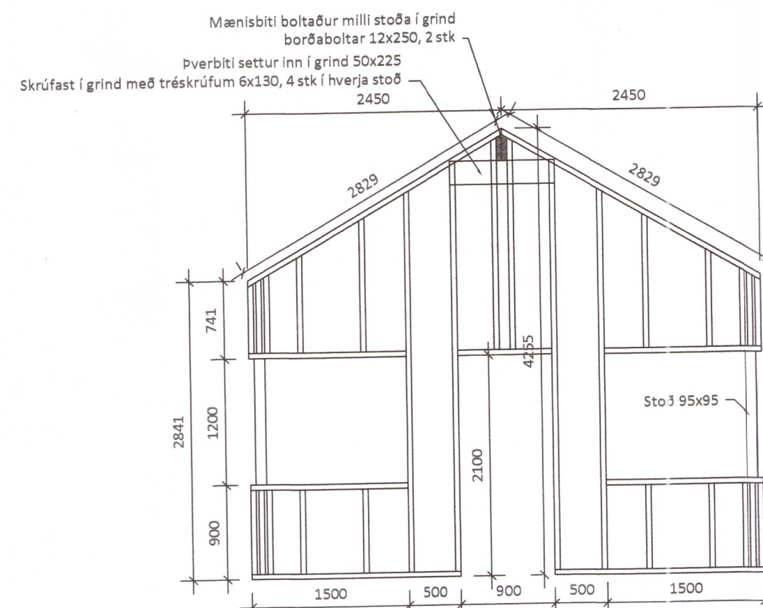
GRIND 5 Mkv. 1:50
