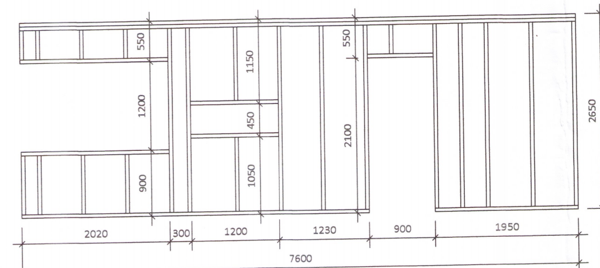
GRIND 4 Mkv. 1:50
