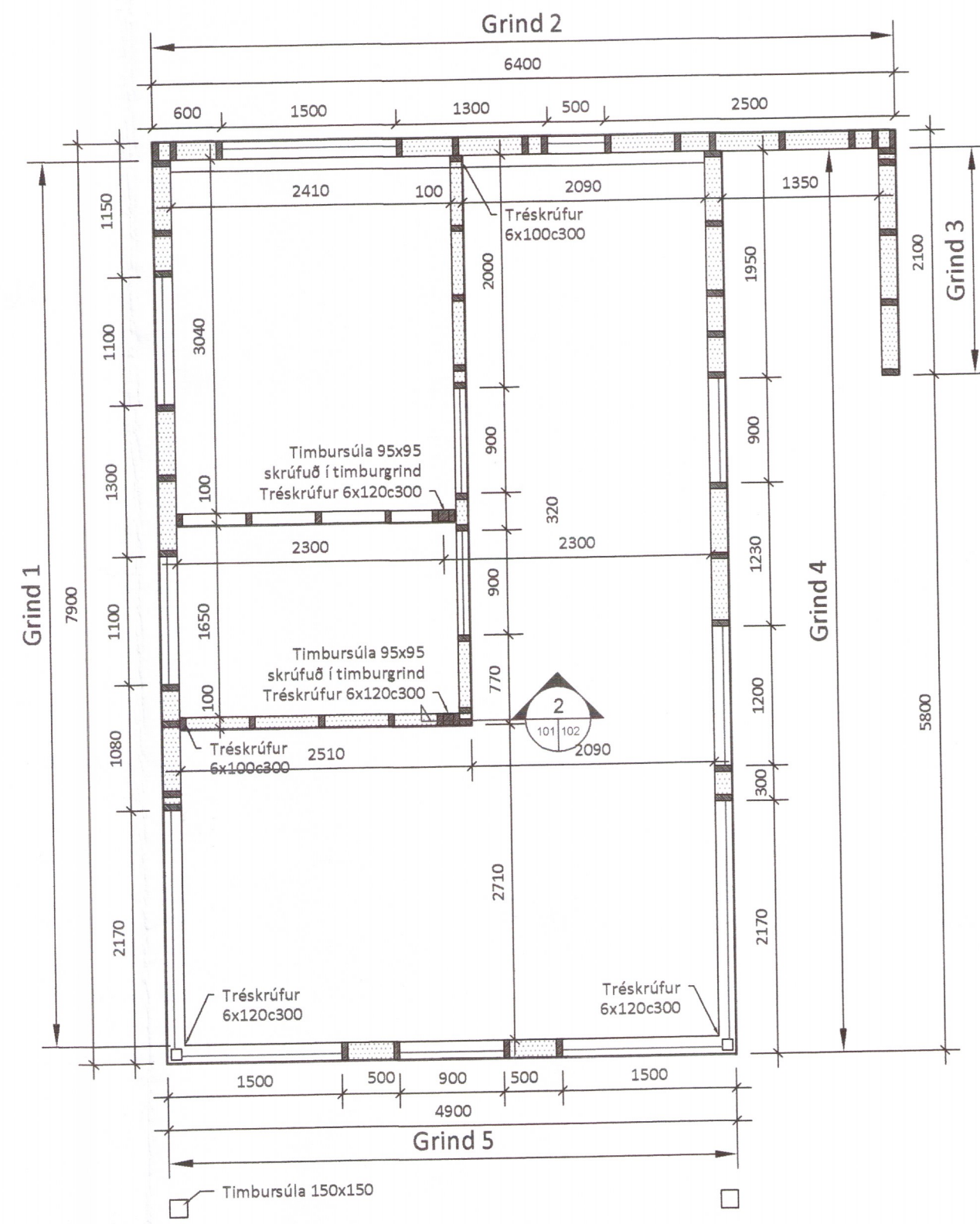
GRUNNMYND-VEGGIR Mkv. 1:50
