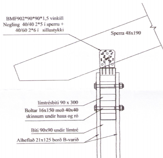
201 FESTING SPERRU VIÐ LÍMTRÉSBITA 202|204 Mkv: 1/10
