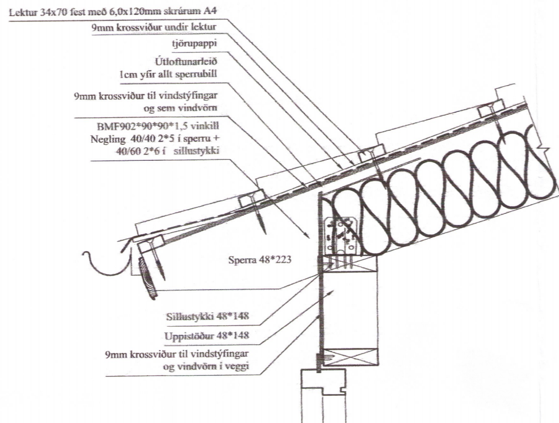
202 FESTING SPERRU VIÐ ÚTHLÍÐAR 202|204 Mkv: 1/10
