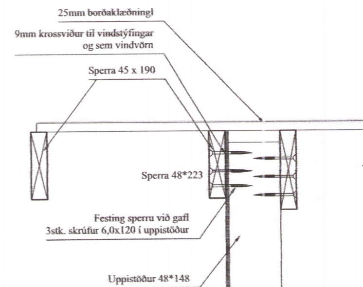
204 FRÁGANGUR VIÐ GAFLA 202|204 Mkv: 1/10
