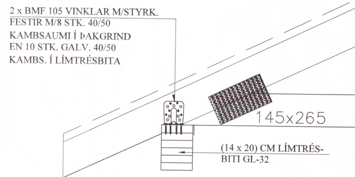
C4 SNIÐ. 1:10 1-04
