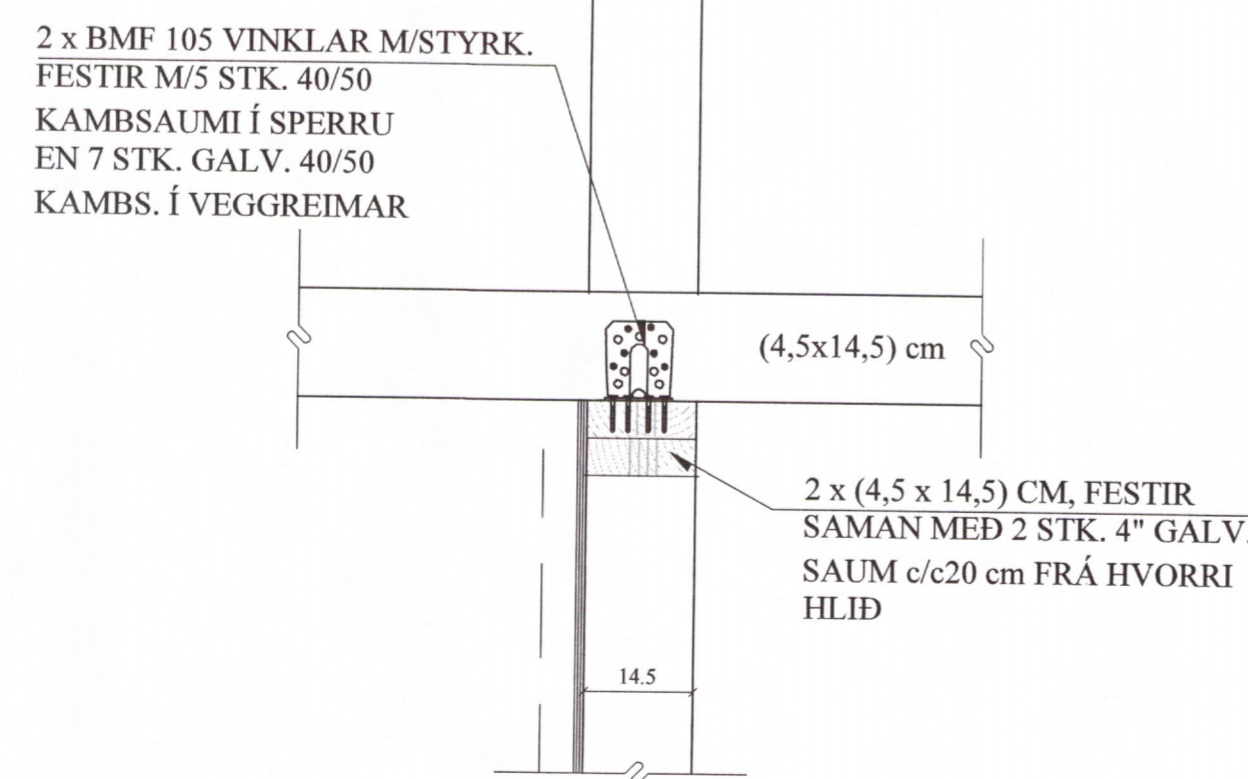
D4 SNIÐ. 1:10 1-04
