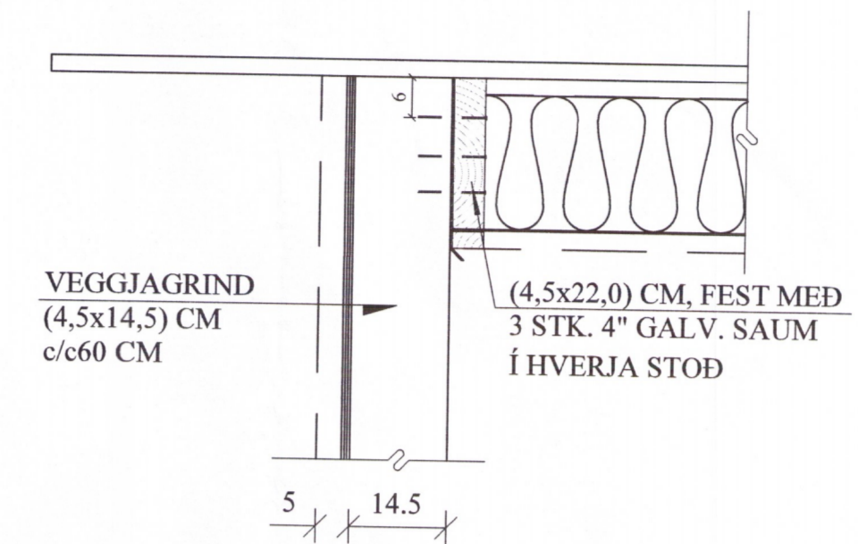
S2 SÚLA. 1:10 1-04
