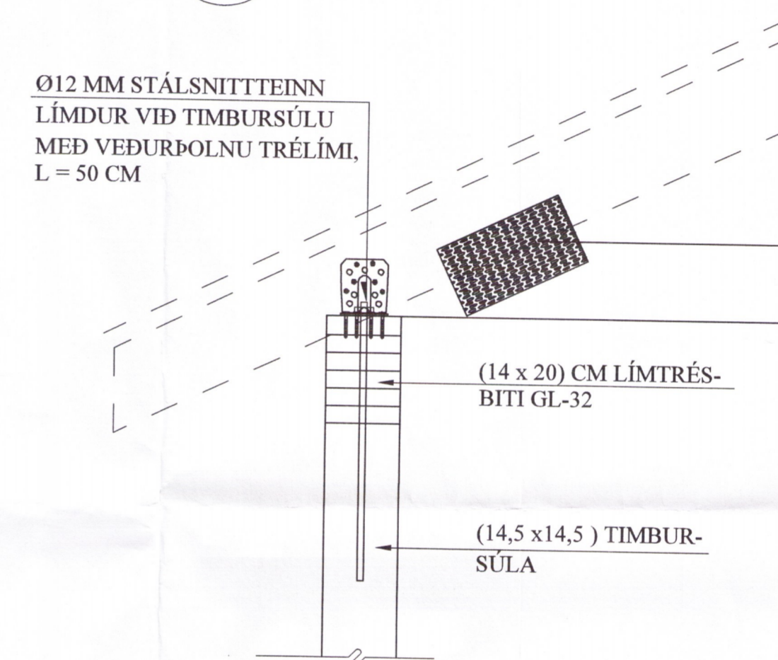
S2 SÚLA. 1:10 1-04
