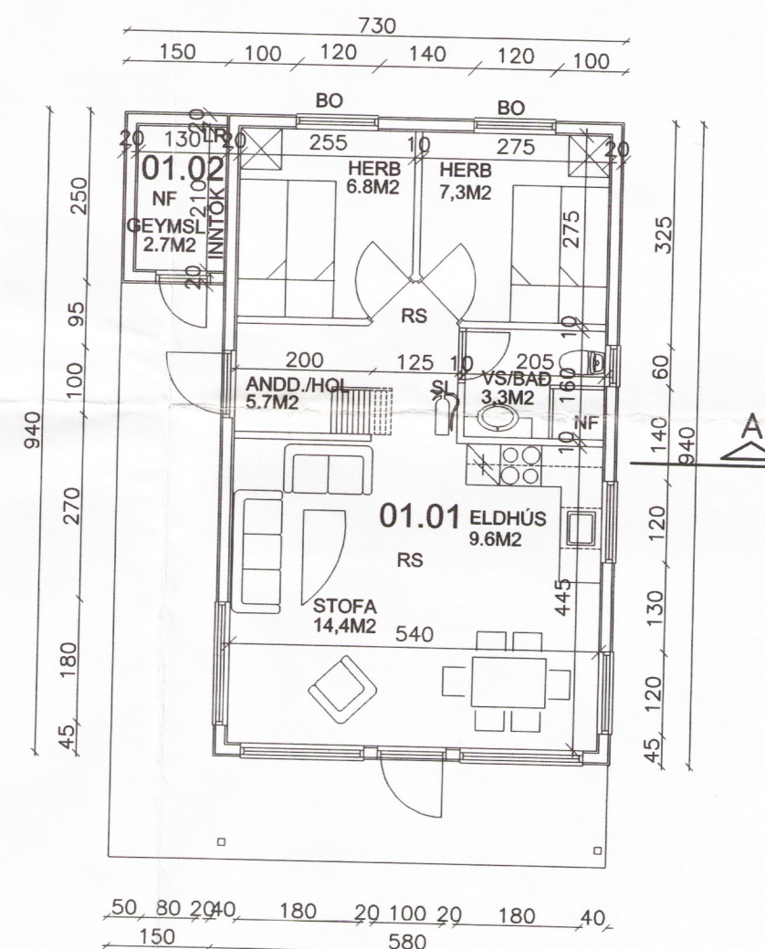
GRUNNMYND
