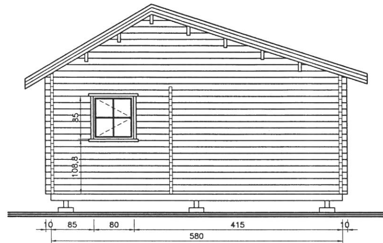
Norðurhlið. Mkv.1:50
