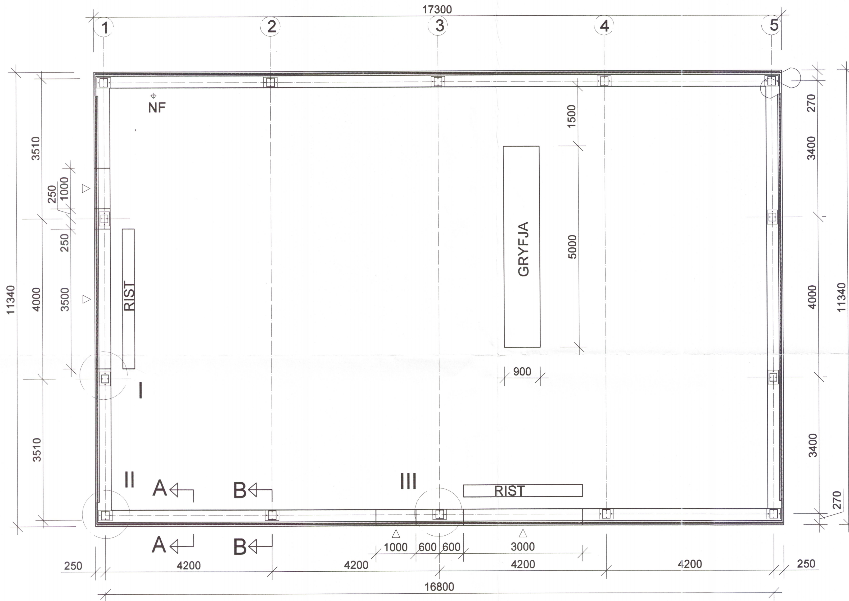
GRUNNMYND 1:50
