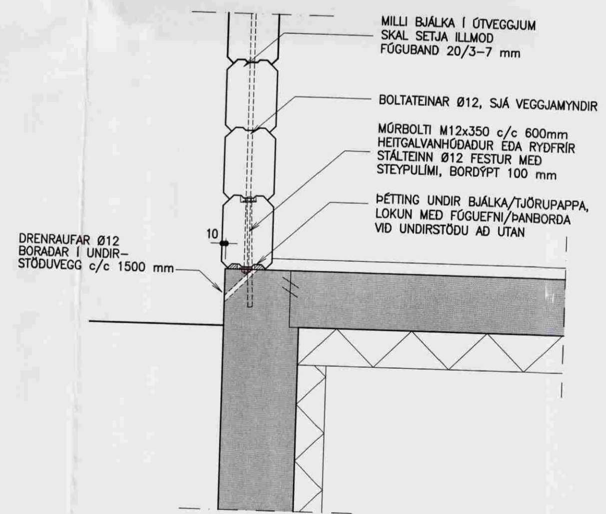
FESTING BJÁLKAVEGGS ADALHÚSS VID UNDIRSTÖÐU 1:10
