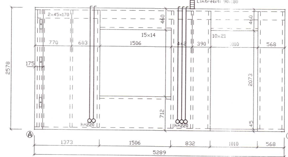
VEGGEINING E8 1:50
