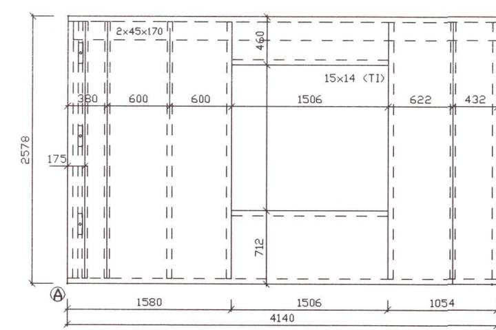
VEGGEINING E3 1:50
