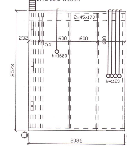
VEGGEINING E9 1:50
