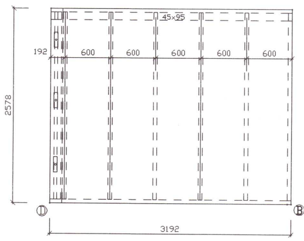
VEGGEINING E7 1:50
