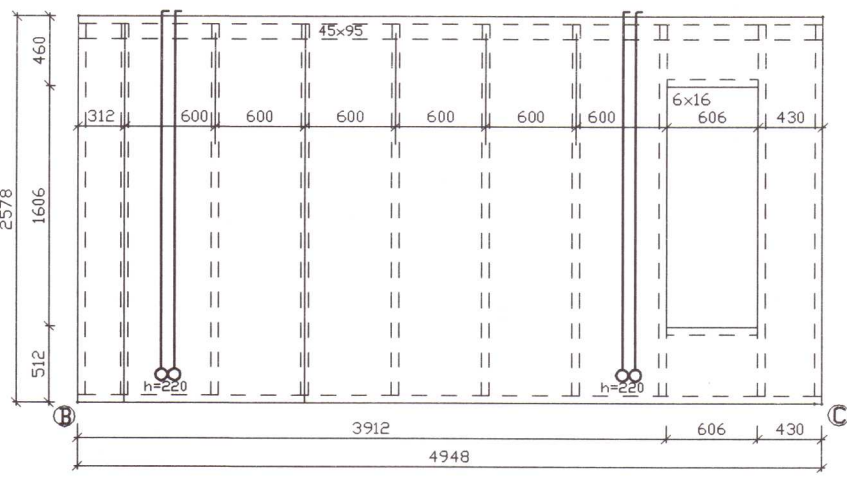
VEGGEINING E1 1:50
