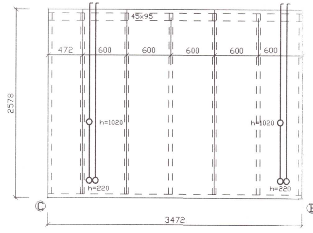
VEGGEINING E2 1:50
