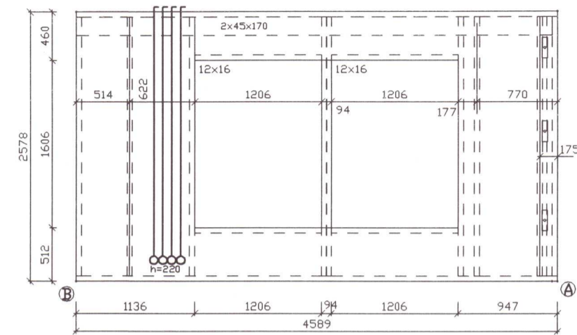
VEGGEINING E10 1:50
