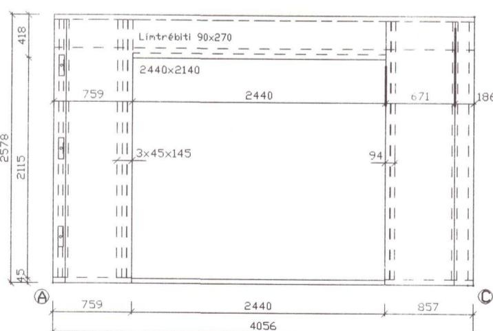
VEGGEINING E17 1:50
