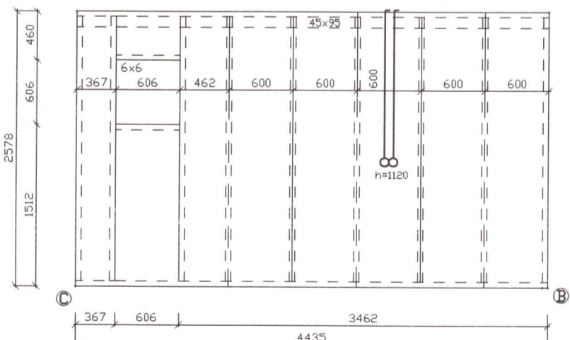
VEGGEINING E16 1:50
