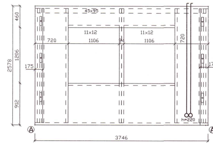
VEGGEINING E12 1:50
