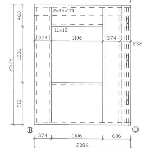
VEGGEINING E11 1:50
