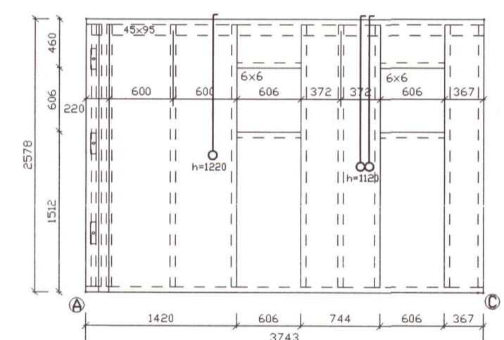
VEGGEINING E15 1:50
