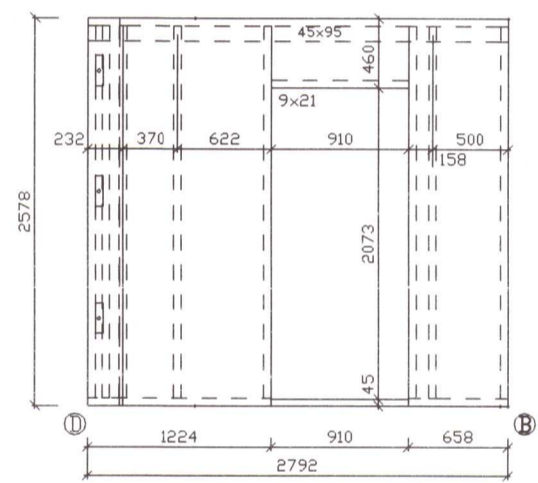
VEGGEINING E13 1:50
