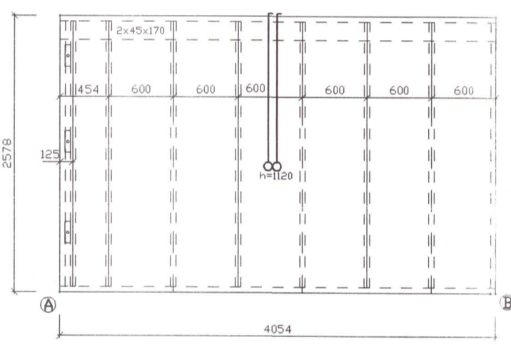
VEGGEINING E14 1:50
