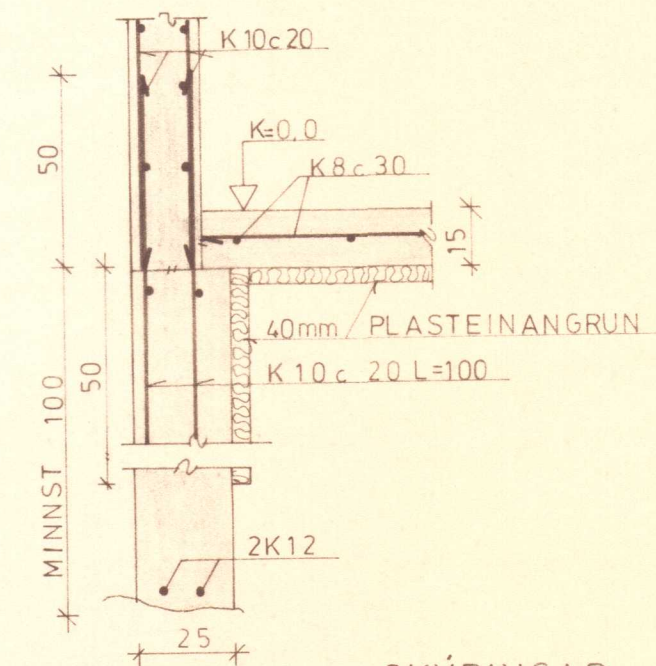
SNIÐ I-I
