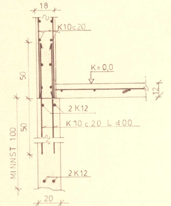
SNIÐ J-J
