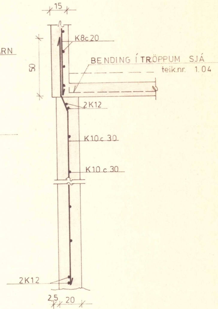
SNIÐ F-F
