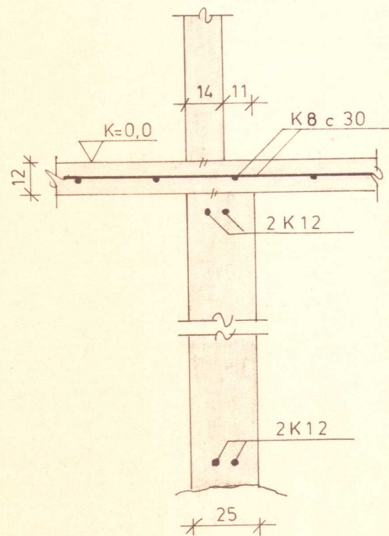
SNIÐ D-D
