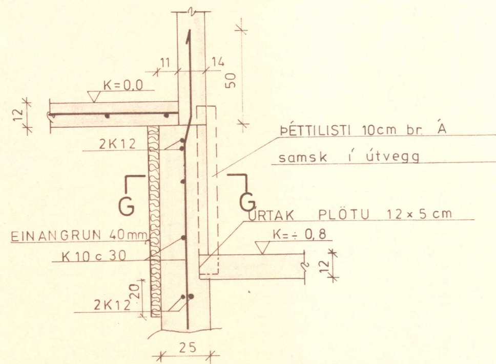
SNIÐ E-E
