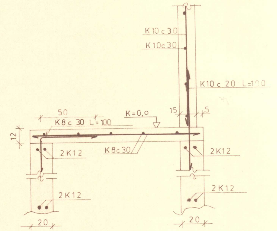
SNIÐ H-H
