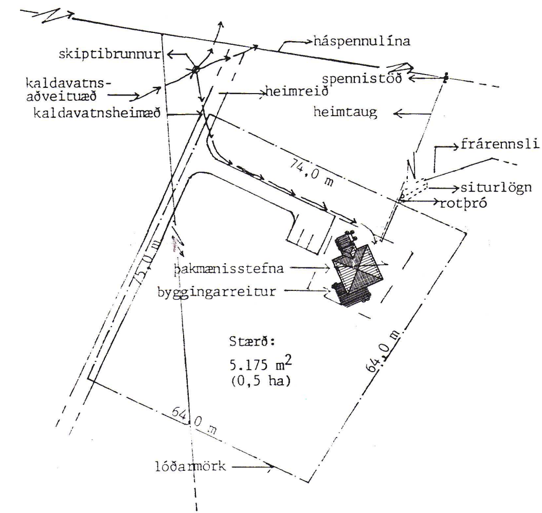
AFSTÖÐUMYND M. 1:1000
