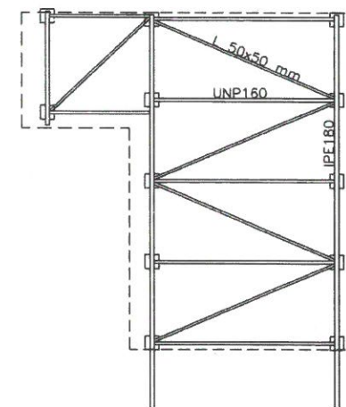
UNDIRSTÖÐUR 1:100
