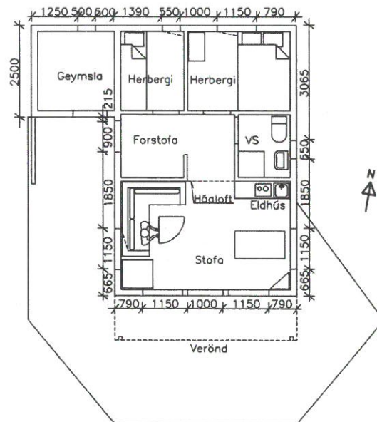
GRUNNMYND 1:100
