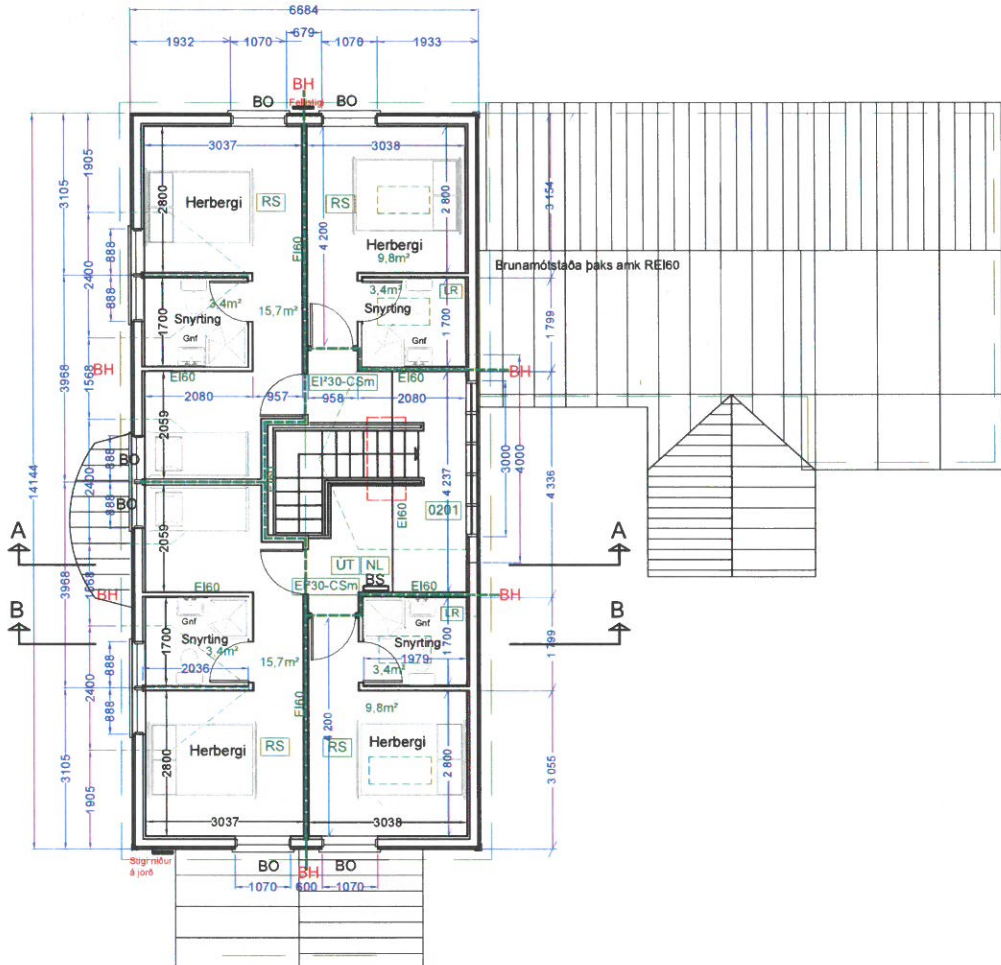
GRUNNMYND 2.HÆÐ
