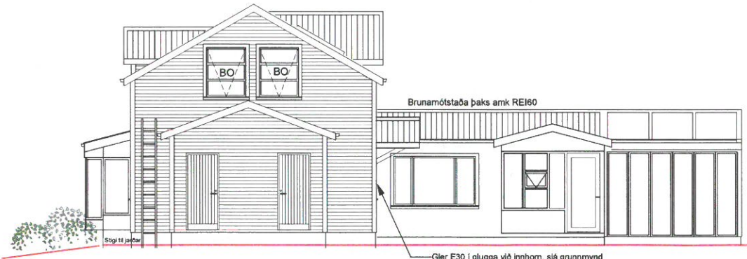
SUDVESTURHLIÐ, 1:100
