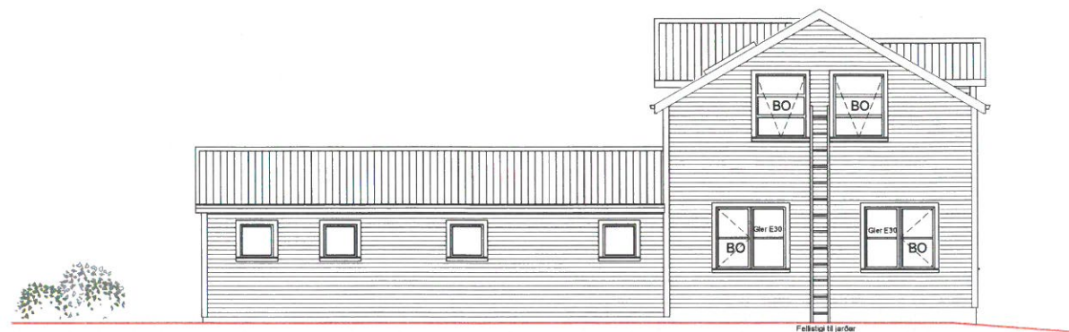
NORÐAUSTURHLIÐ, 1:100
