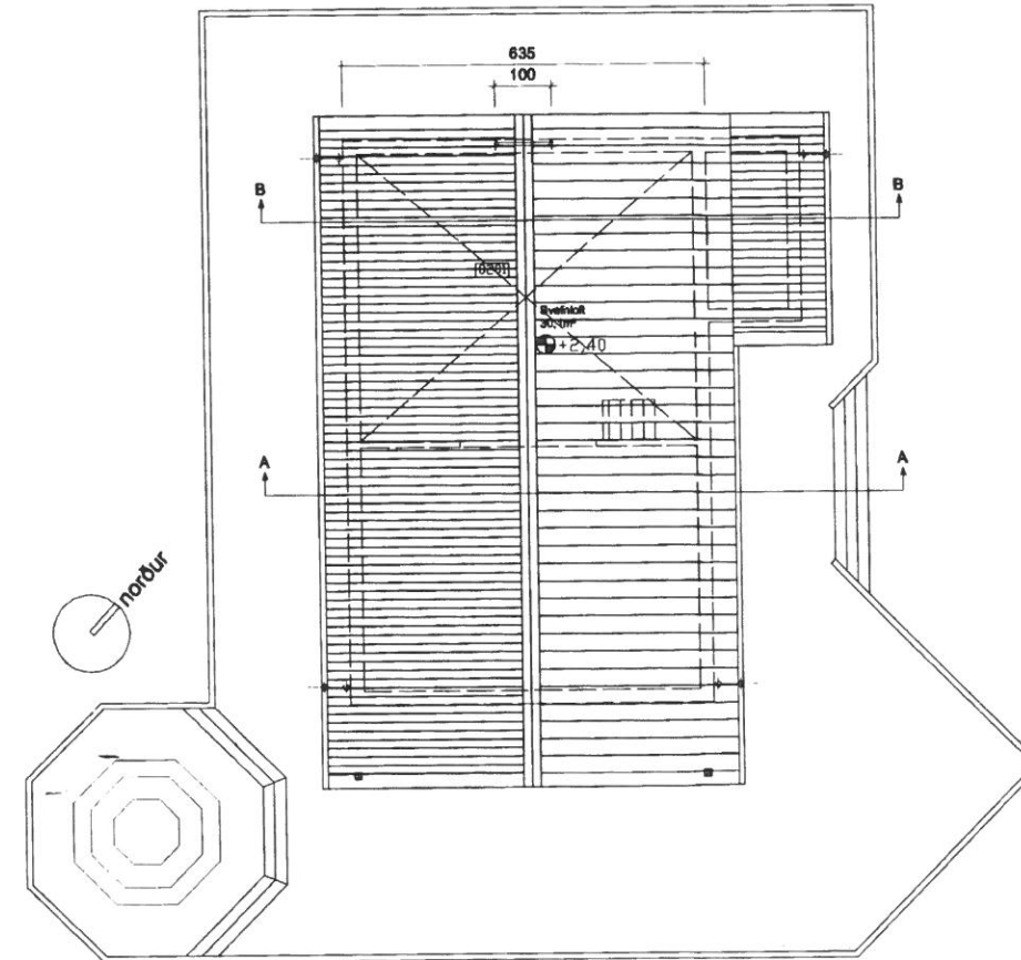
Þakmynd (ásamt grunnmynd svefnlofts)
