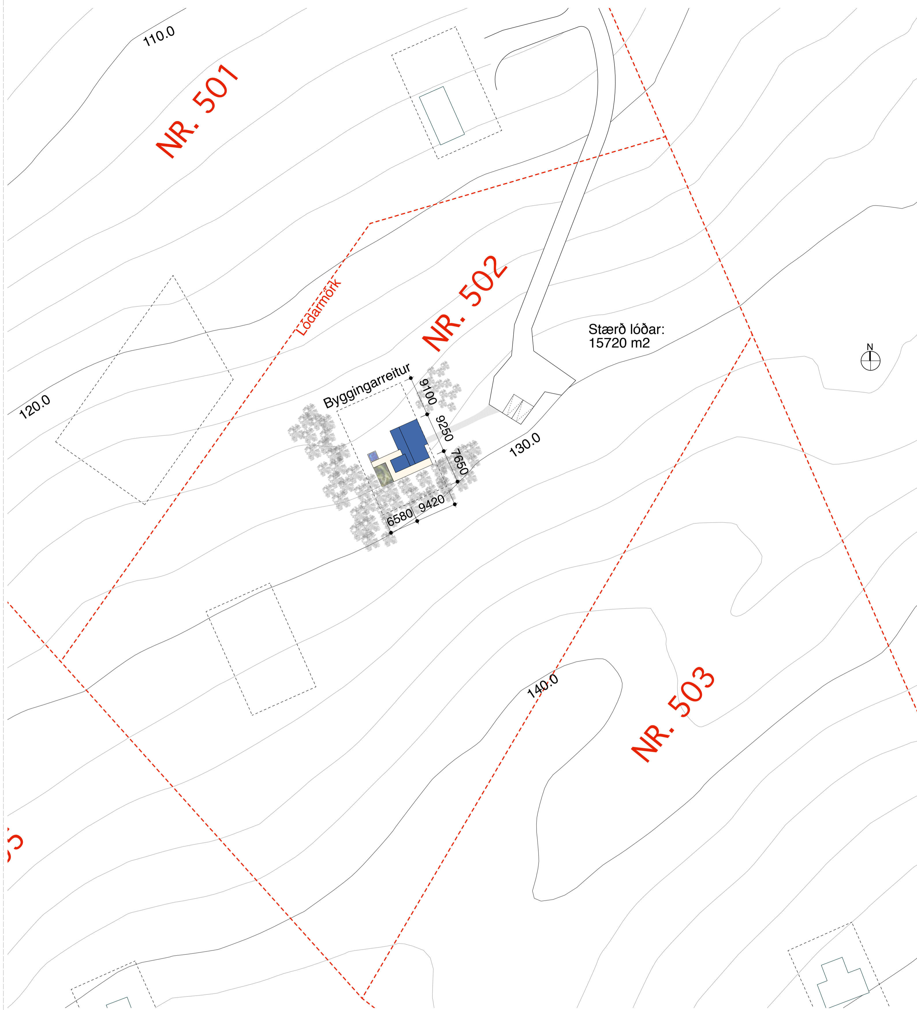
AFSTÖÐUMYND MKV. 1:500
