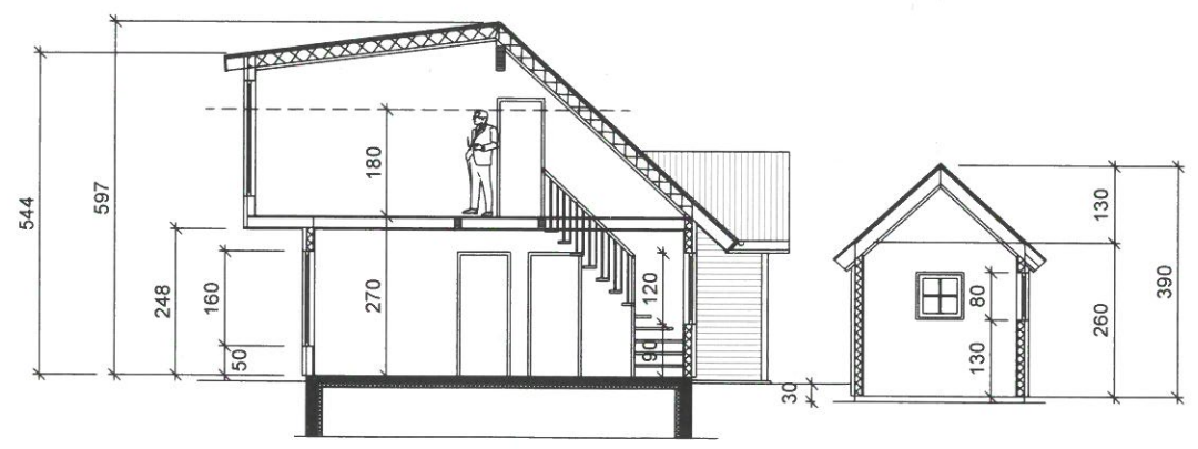
SNIÐ A-A
