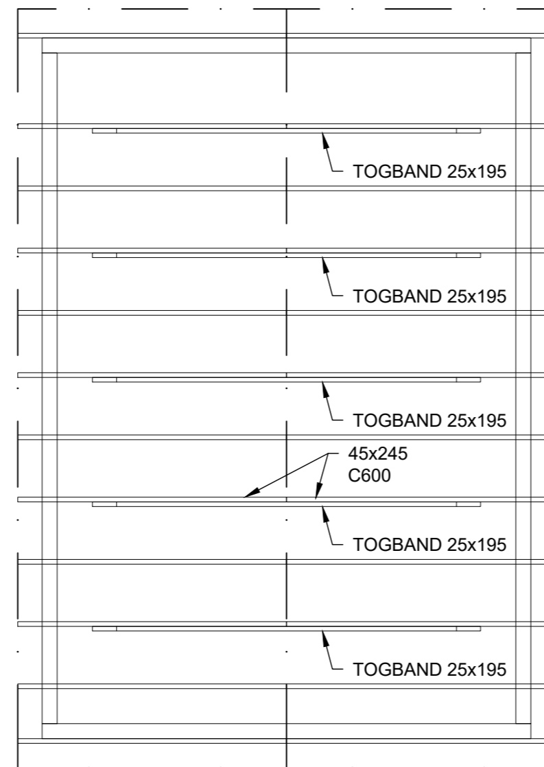
ÞAKSPERRUR 1:50 (A2)
