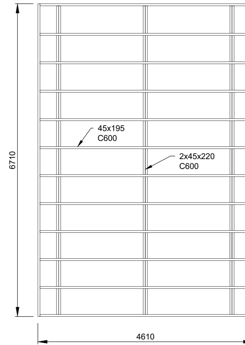
GÓLFBITAR 1:50 (A2)
