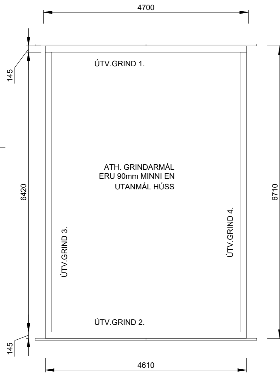
ÚTV.GRINDUR GRUNNMYND 1:50 (A2)
