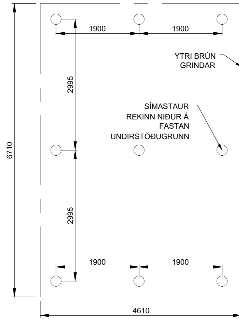
STAURAR 1:50 (A2)
