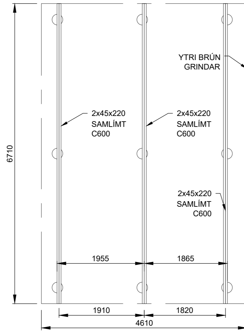
GÓLFDREGARAR 1:50 (A2)
