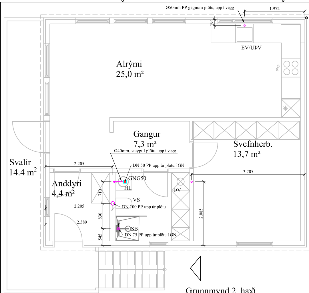
Grunnmynd 2. hæð
