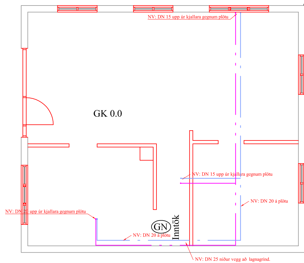
Grunnmynd kjallari/1.hæð
