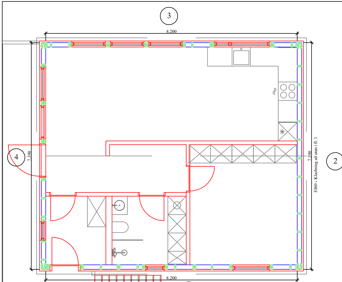
Grunnmynd 2. hæð - veggjagridnur
