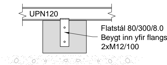
F1 SÉRMYND Mkv. 1:20
