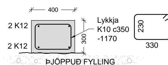
B1 SNIÐ Mkv. 1:20
