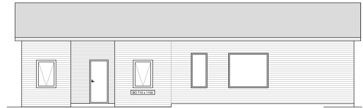
ÚTLIT NORÐUR Mkv. 1:100
