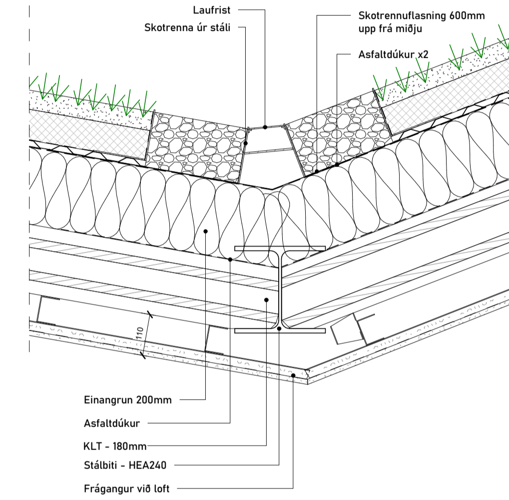
3 LÓ - Frágangur á þaksamskeytum 1 : 10
