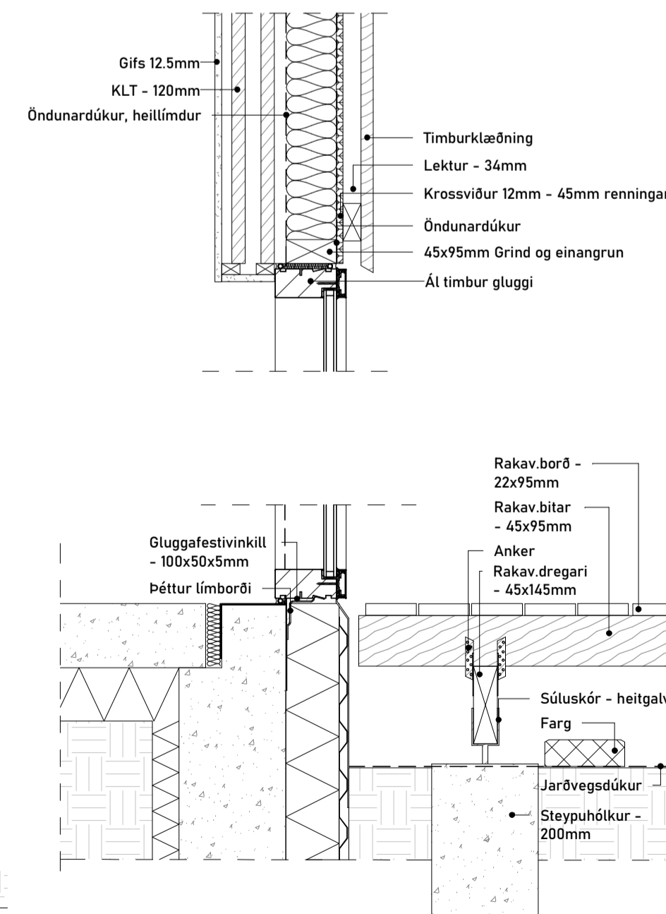
4 LÓ - Frágangur á glugga í borðstofu 1 : 10
