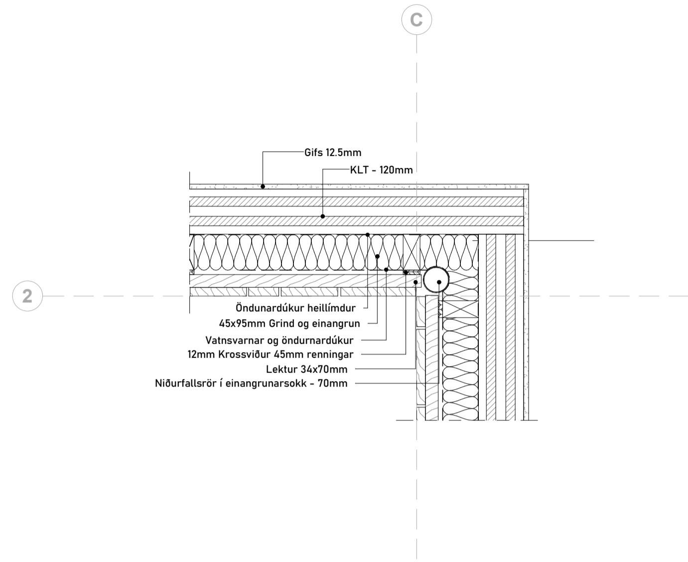
7 LÁ - Frágangur á niðurfalli við horn 1:10
