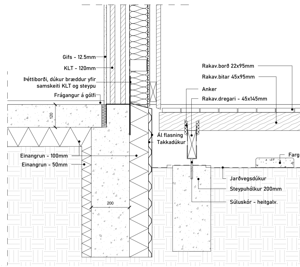
2 LÓ - Frágangur á sökkli við pall 1 : 10
