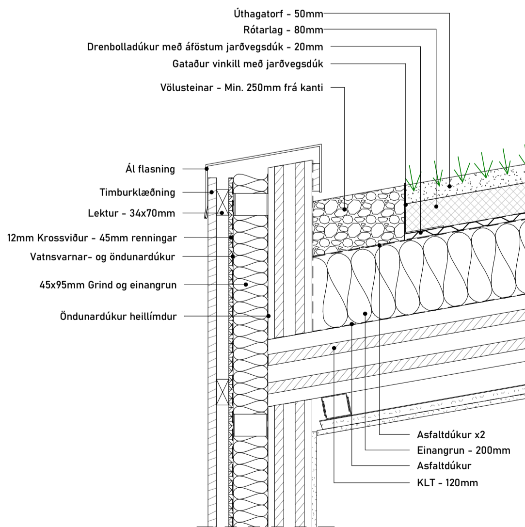
5 LÓ - Frágangur á þakkanti 1 : 10
