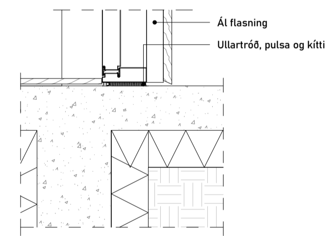
10 LÓ - Frágangur á hurð 1:10
