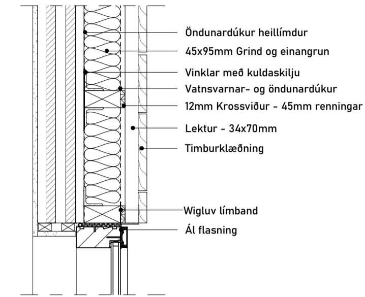
9 LÁ - Frágangur á glugga 1:10
