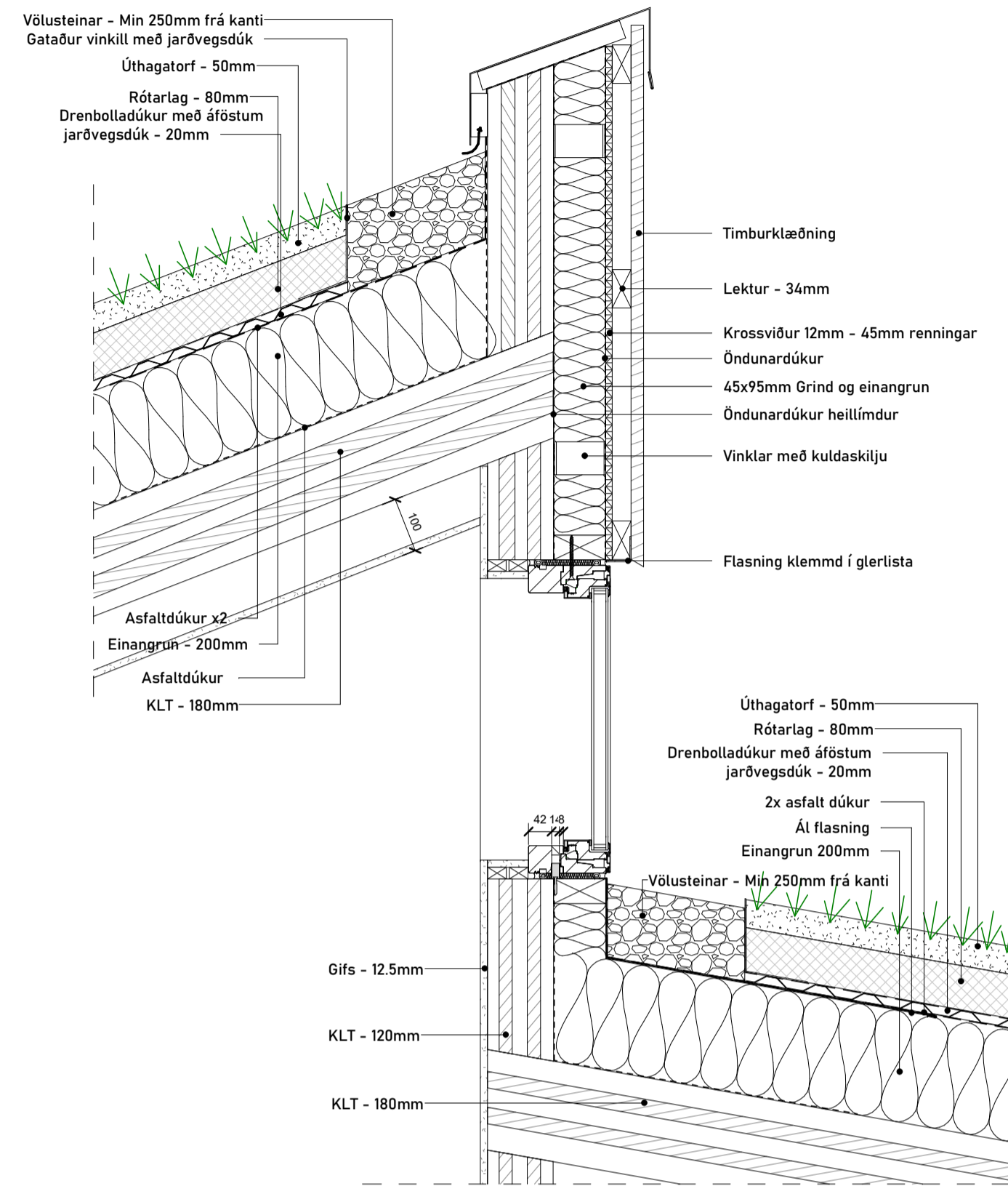
1 LÓ - Frágangur á þakglugga 1 : 10
