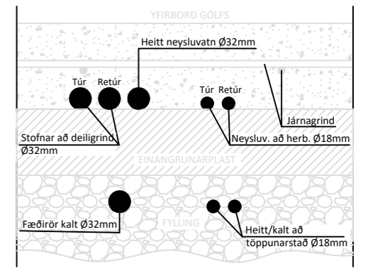
Skýringamynd af gati fyrir ídráttarrör, gólfhita- og neysluvatnslagnir
