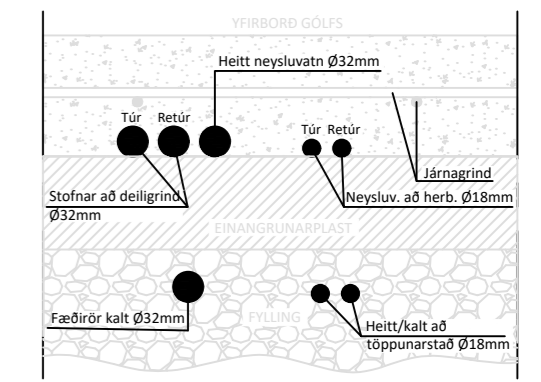
Skýringamynd af gati fyrir ídráttarrör, gólfhita- og neysluvatnslagnir
