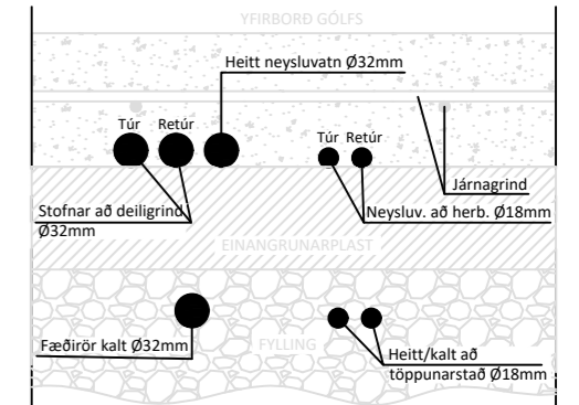
Skýringamynd af gati fyrir ídráttarrör, gólhita- og neyglvatnslagnir
