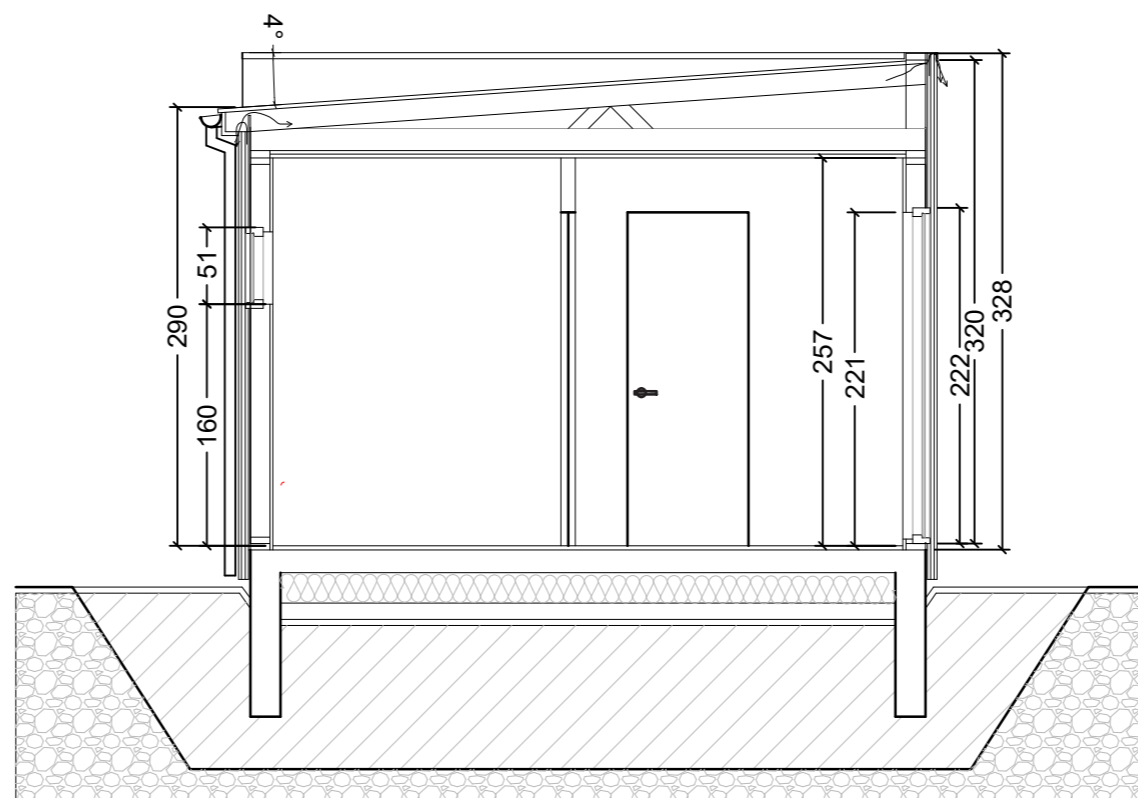
SNIÐ A 1:50
