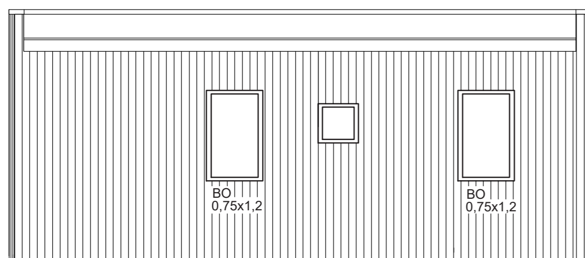
ÚTLIT, AUSTURHLIÐ 1:50
