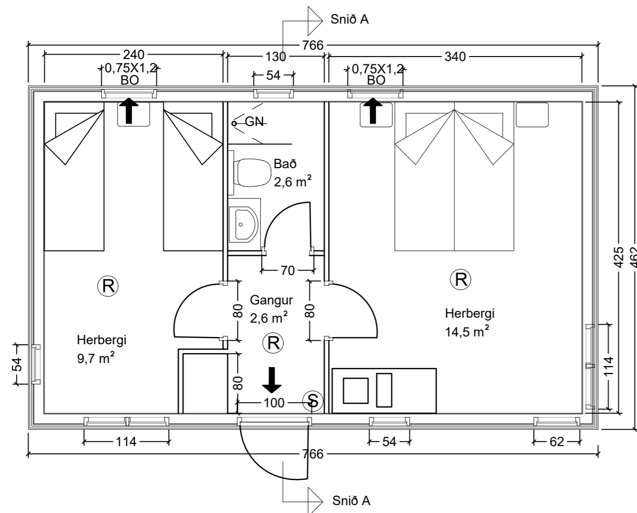
GRUNNMYND 1:50
