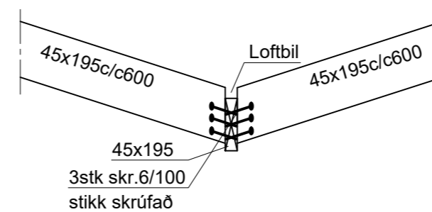
Festing við kverksperu 1:20
