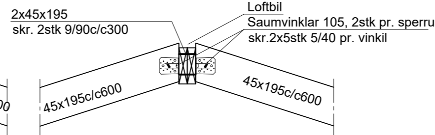
p5 1:20
