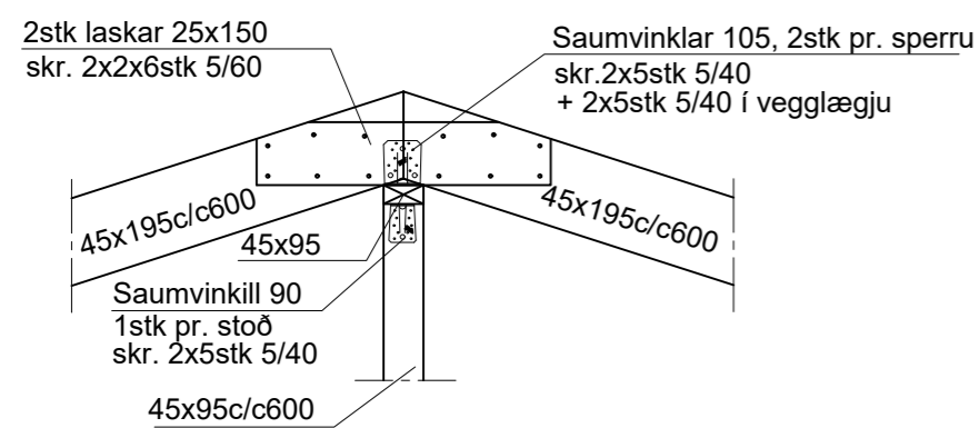
p3 1:20
