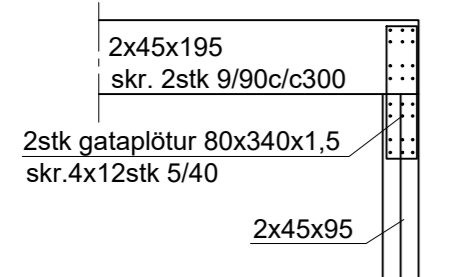
F1 1:20
