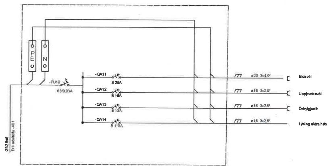
TAFLA -A02 Aðaltafla EINLÍNUMYND Núverandi hús
