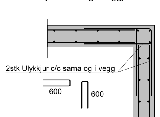
Snið í jámbendingu veggja í úthorni 1:20
