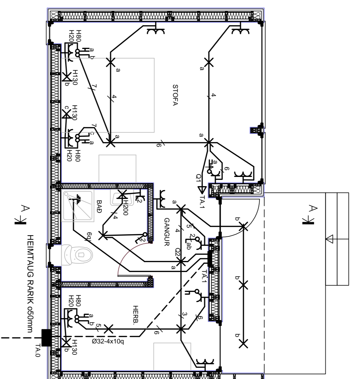
GRUNNMÝND RAFLAGNIR MKV 1:50
