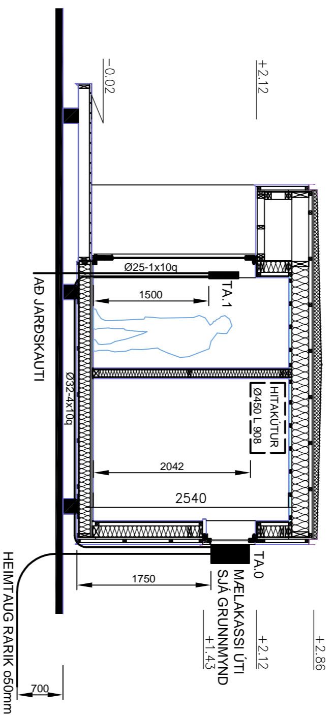
SNEIDING A-A MKV 1:50
