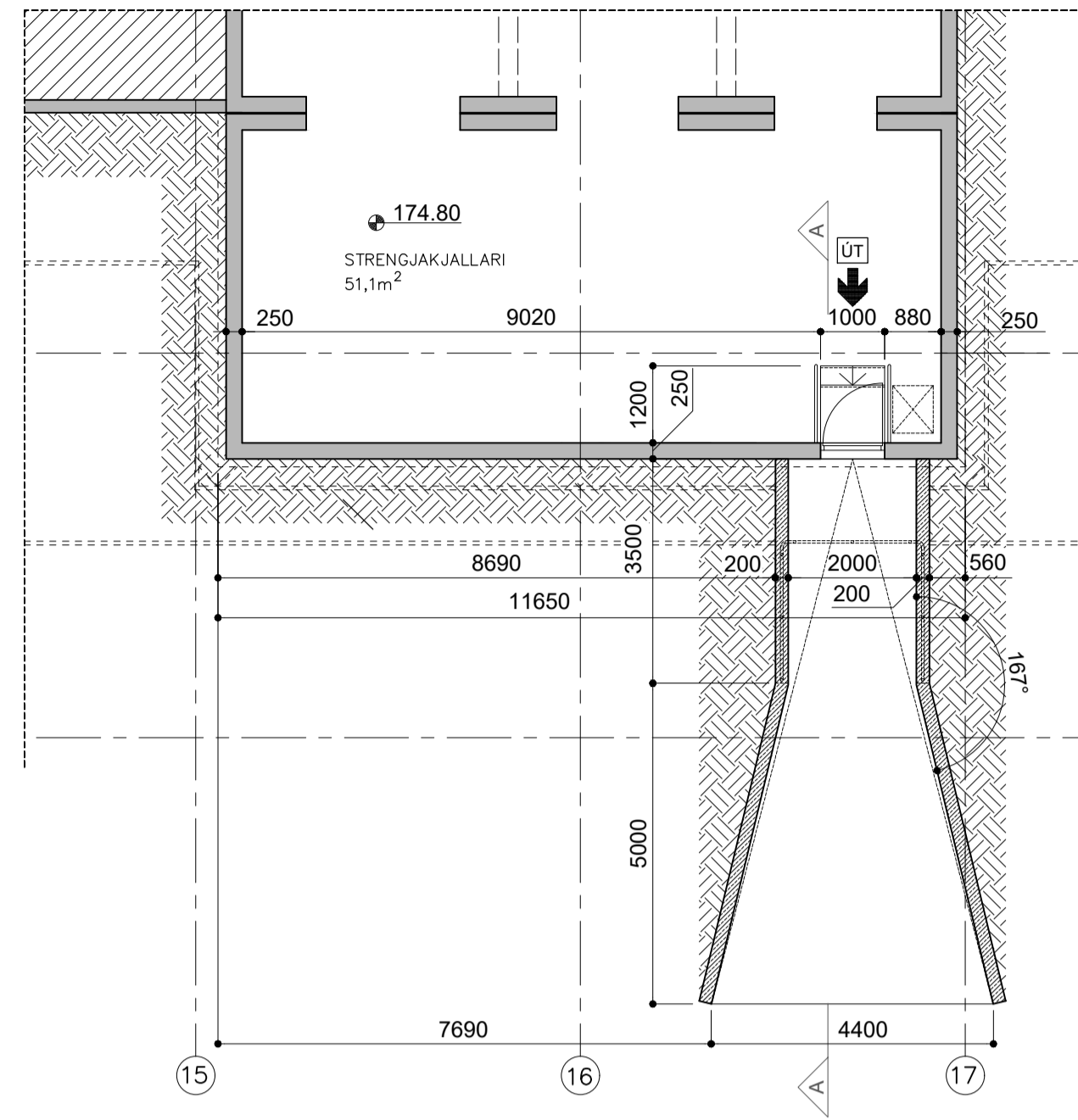
Grunnmynd kjallara mkv 1:100
