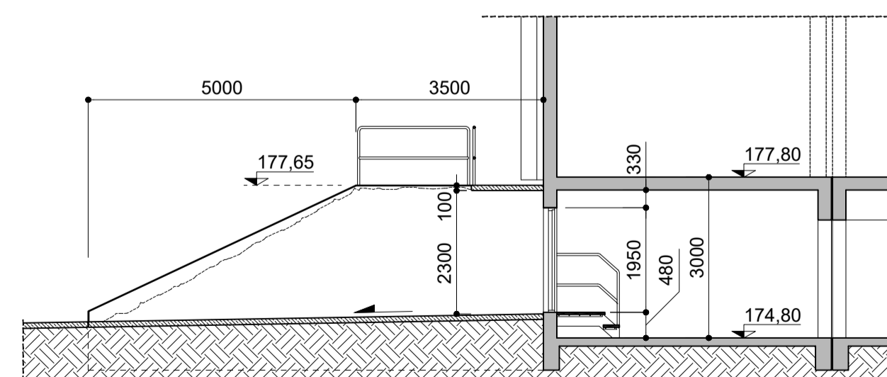
Sneiðing A-A mkv 1:100
