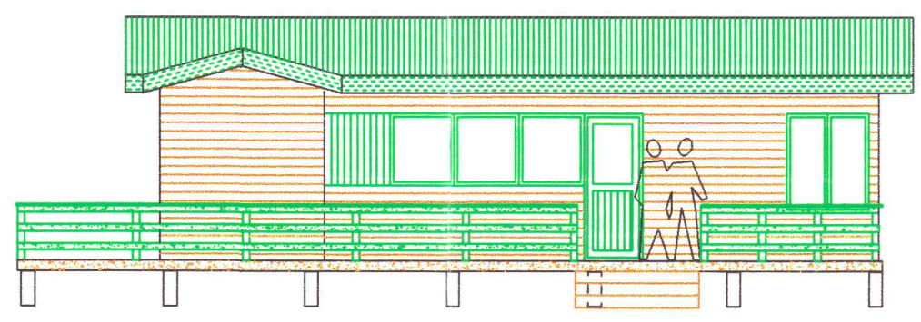
Útlit norðvestur
