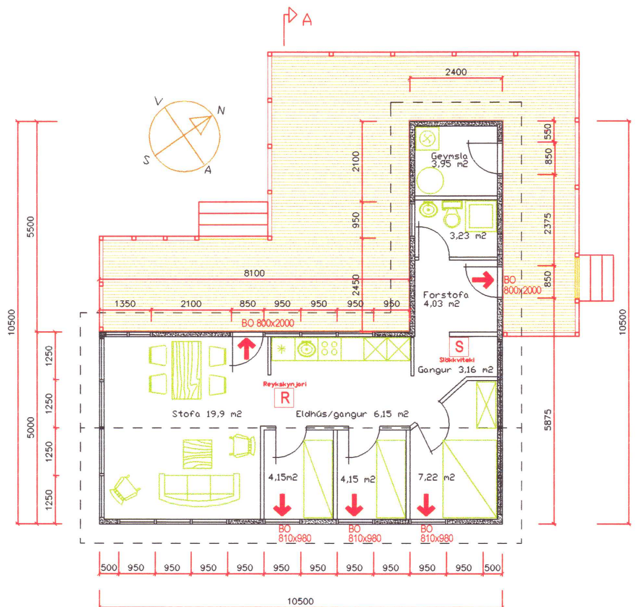
Grunnmynd 1:100
