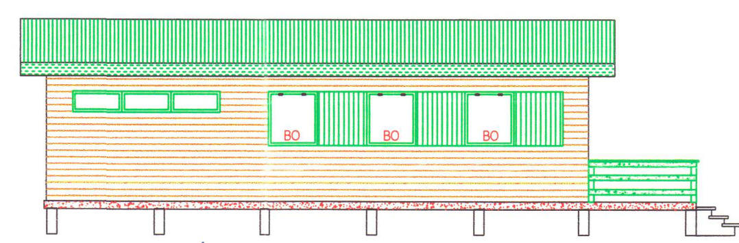
Útlit suðaustur
