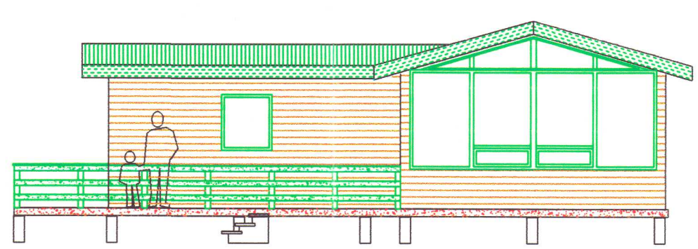
Útlit suðvestur
