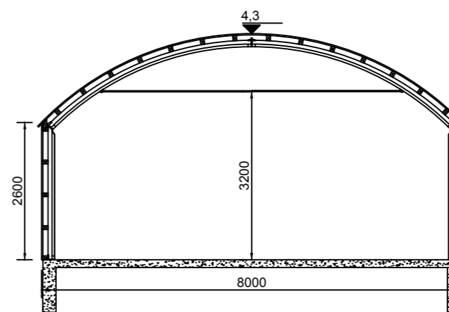
Sneiðing Mkv. 1:100
