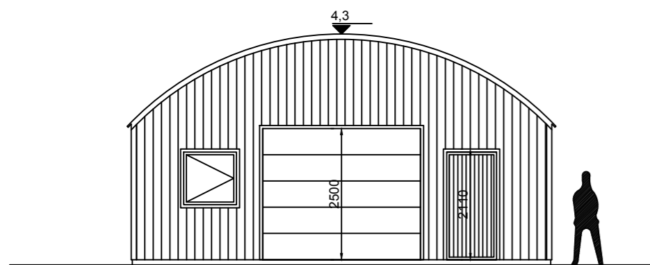
Gafi Mkv. 1:100
