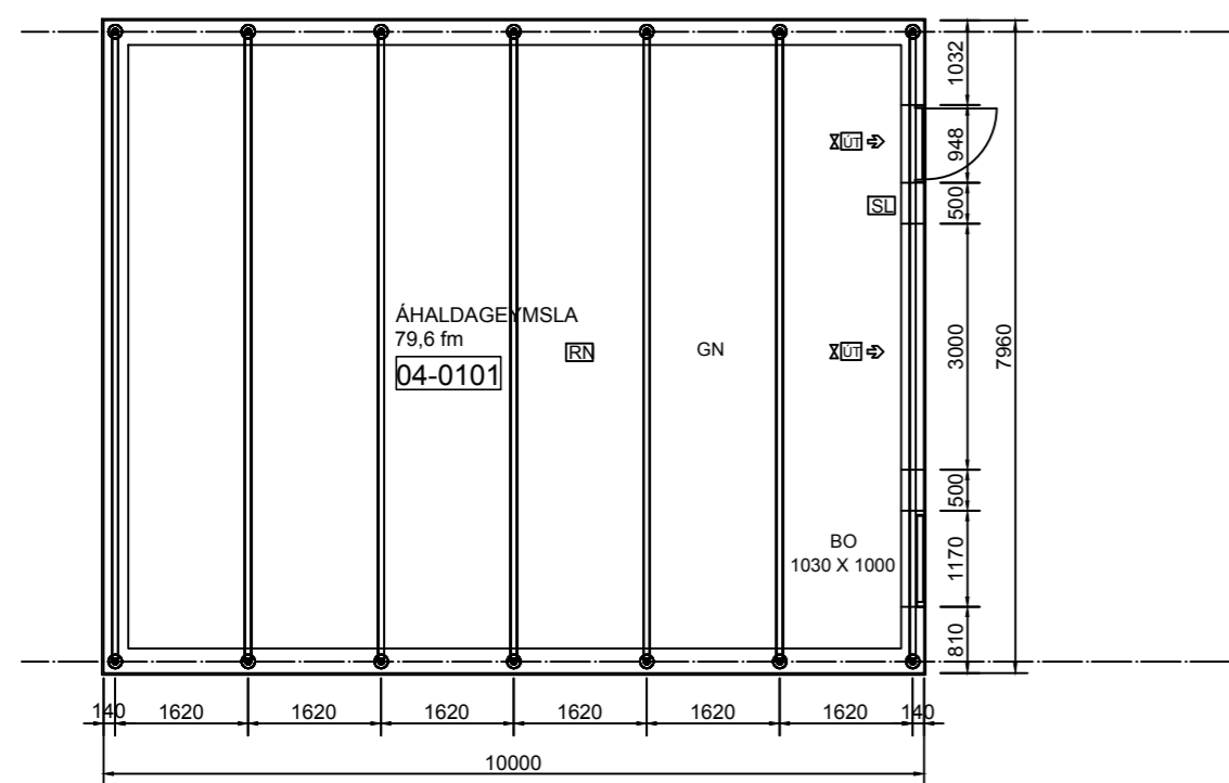
Grunnmynd Mkv. 1:100
