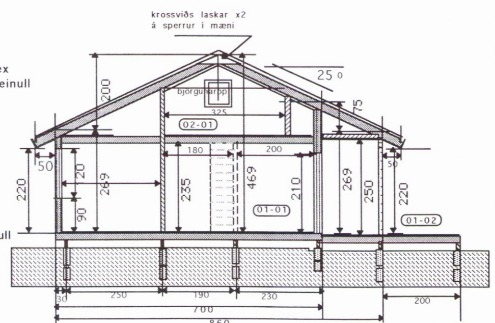
SNID A-A
