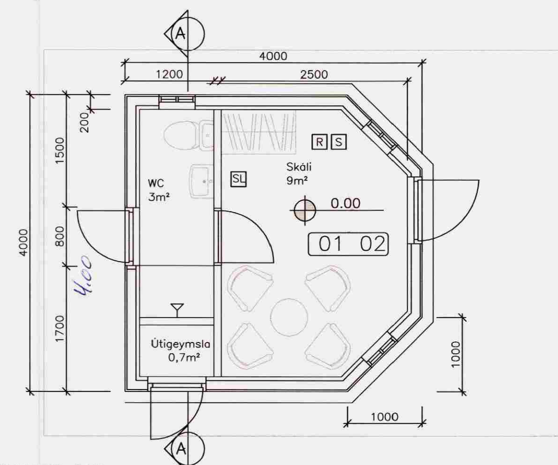
GRUNMYND 1:50
