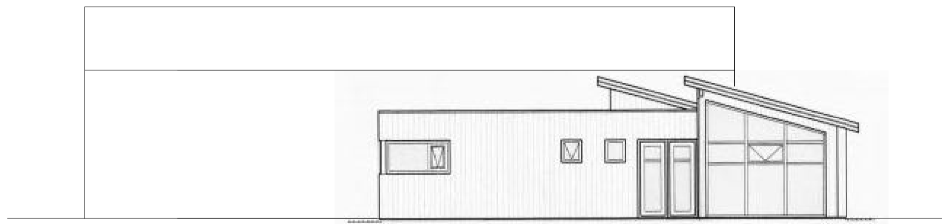
VESTURHLIÐ mkv. 1:100
