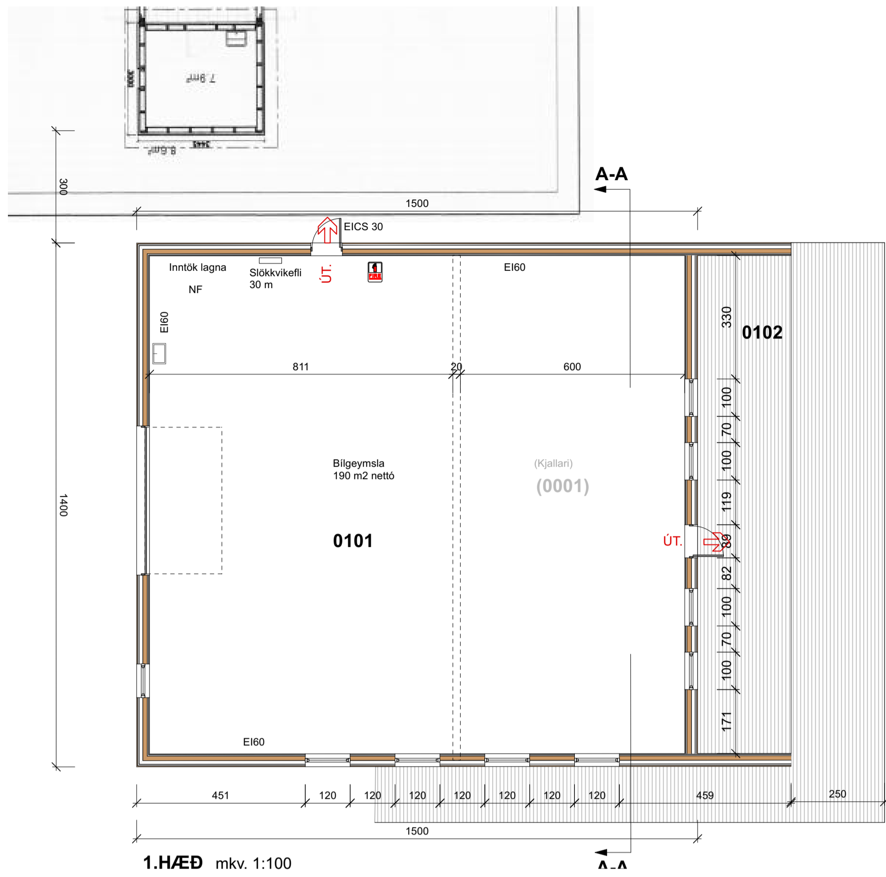
1.HÆÐ mkv. 1:100
