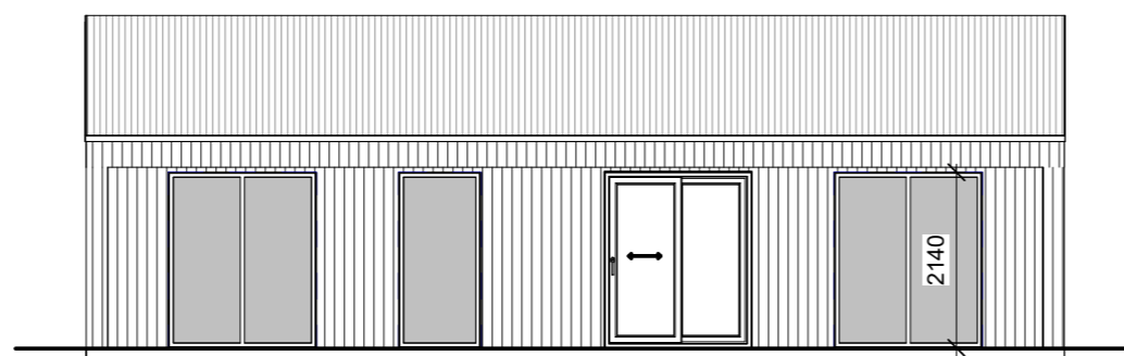
Suður 1: 100
