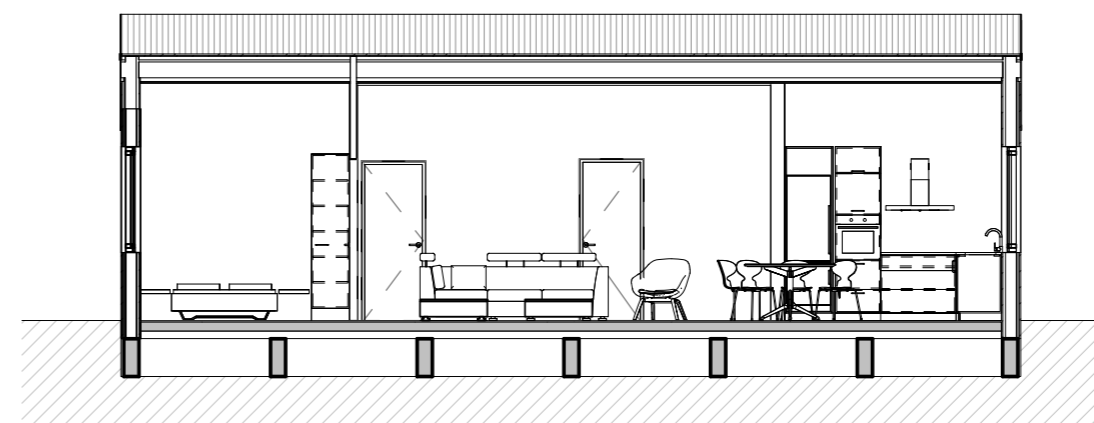
Snið 8 1: 100
