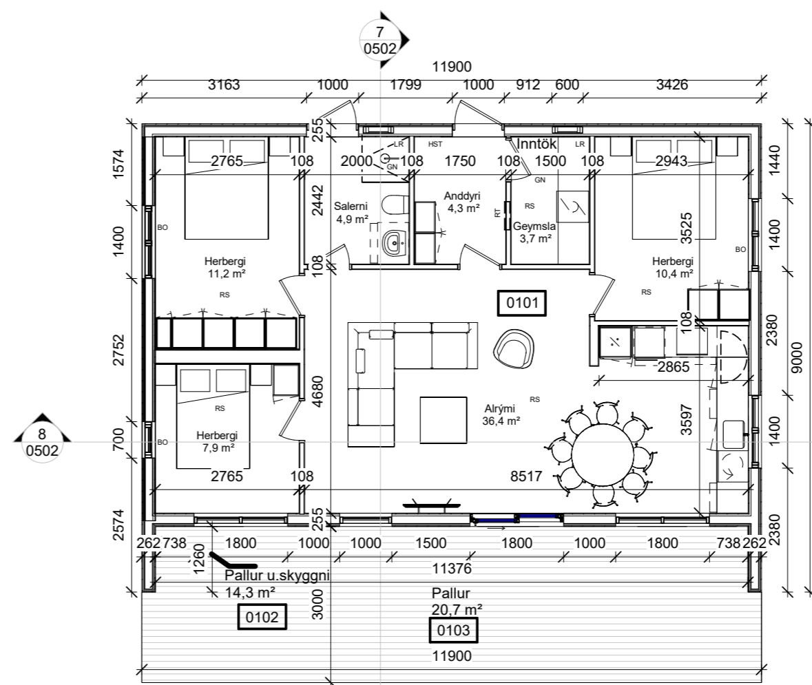
Grunnmynd BN 1: 100
