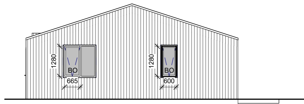
Vestur 1: 100
