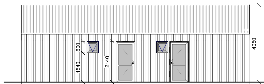
Norður 1: 100
