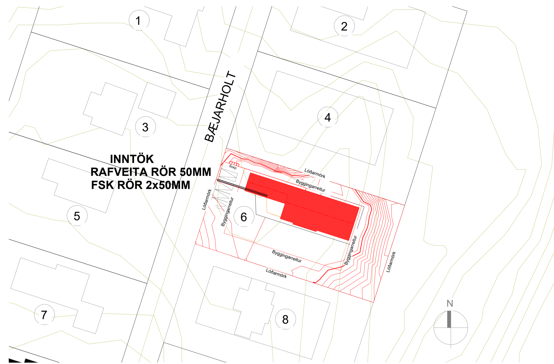
Afstöðumynd 1:500
